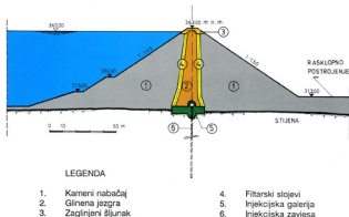
Slika 1. Presjek brane
