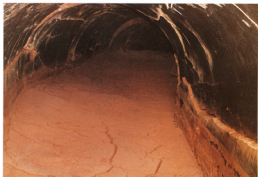
Djelomično razorena injekcijska galerija s nataloženim glinenim materijalom
