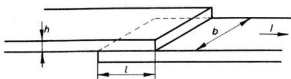
Sl. 306. Preklopni spoj vodiča
