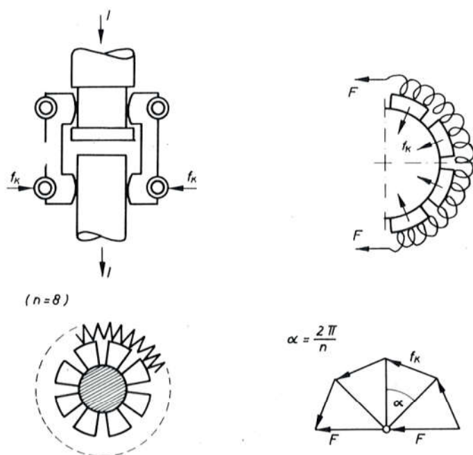
Sl. 314. Pritisak na segmentima tulipanskoga kontakta
