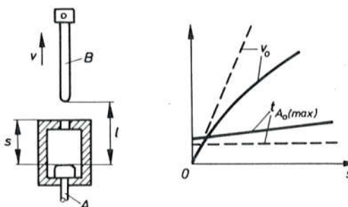
Sl. 718. Optimalna brzina isklapanja
