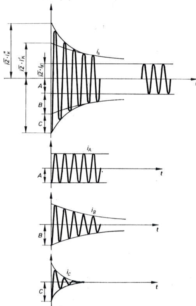
Sl. 6053. Komponente simetrične struje kratkog spoja
