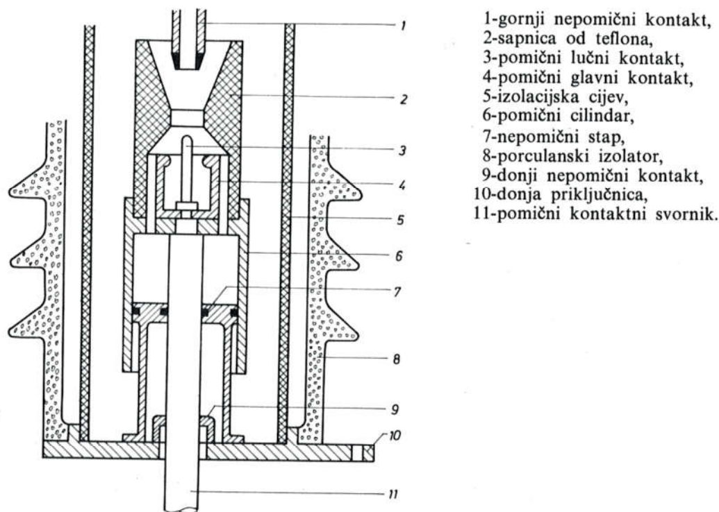
Sl. 754. Autopneumatska komora prekidača s plinom \text{SF}_6
