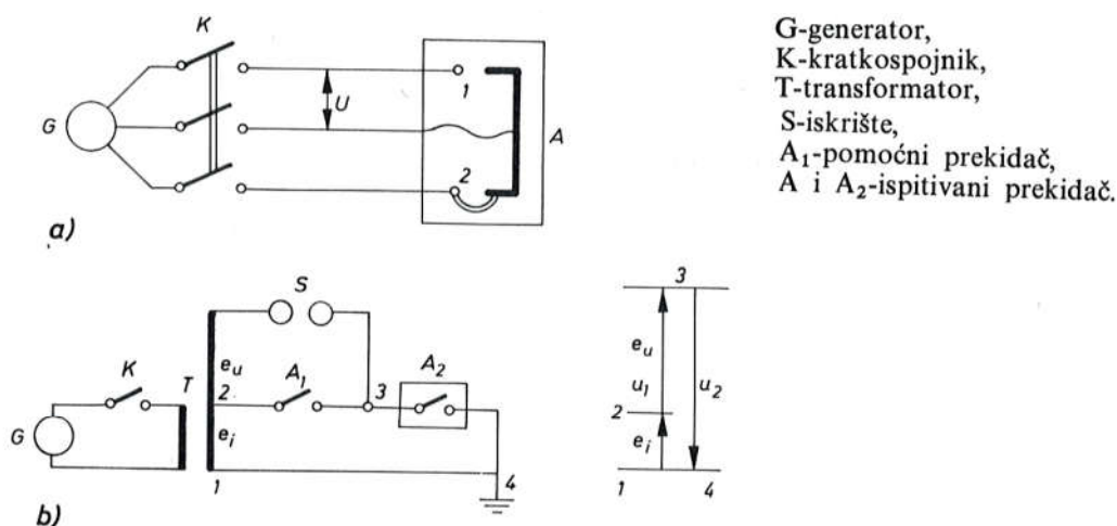
Sl. 771. Ispitni krugovi po Biermannsu (a) i Skeatsu (b)
