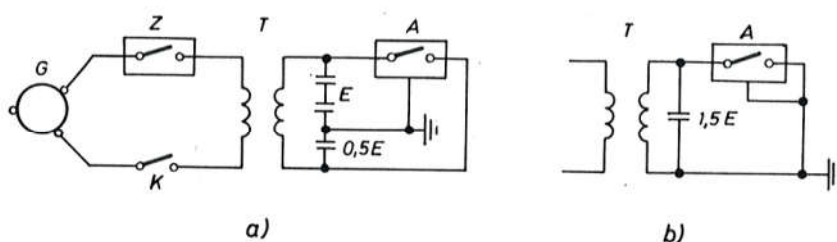
Sl. 767. Jednopolno ispitivanje prekidne moći za mreže s uzemljenim zvjezdištem (a) i za mreže s izoliranim zvjezdištem (b)
