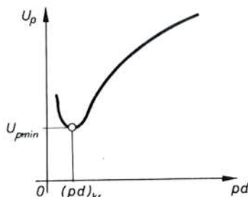
Sl. 412. Grafički prikaz Paschenova zakona
