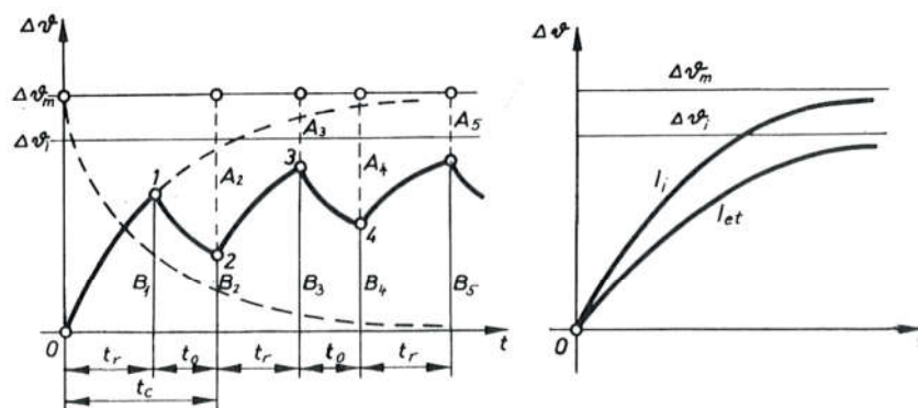
Sl. 308. Zagrijavanje u intermitiranom pogonu
