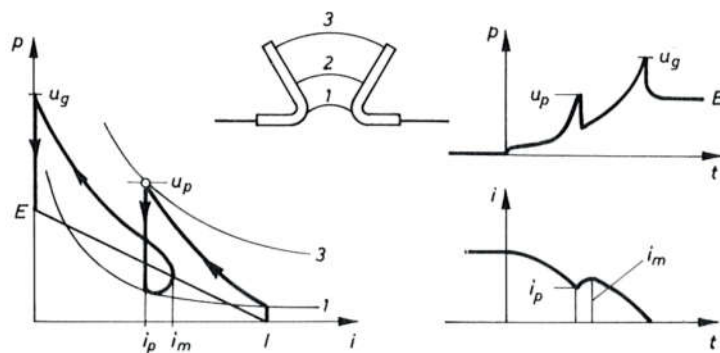
Sl. 6100. Pojave pri gašenju luka među kontaktnim rogovima
