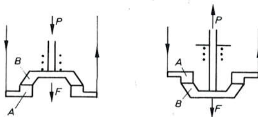
Sl. 510. Utjecaj rasporeda kontaktnog sistema na djelovanje elektrodinamičkih sila
