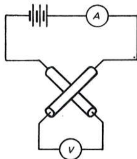
Sl. 204. Mjerenje provlačnog otpora prema formuli (2006)
