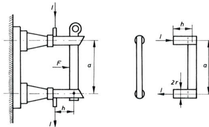
Sl. 504. Određivanje sila na nožu rastavljača
