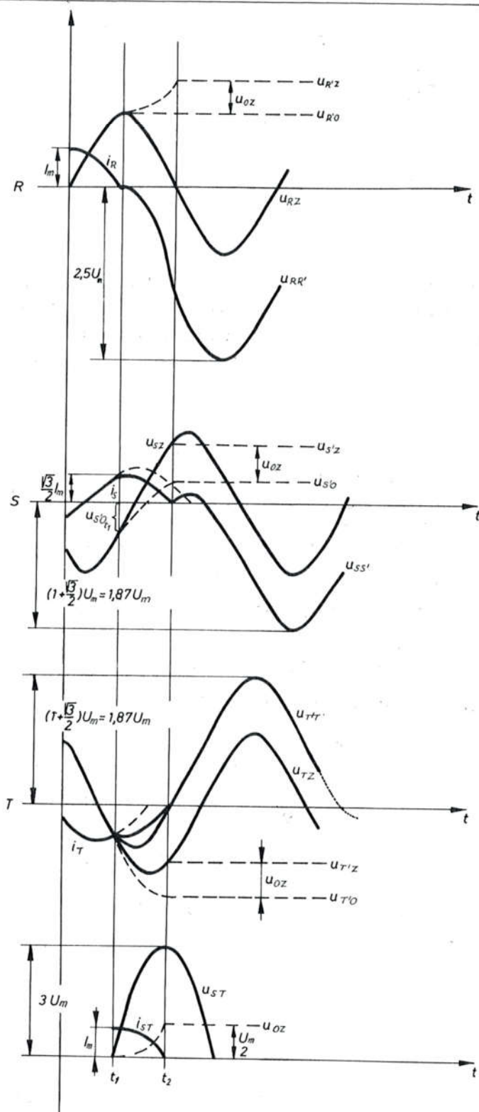
Sl. 6066. Tropolno isklapanje neopterećenih kabela
