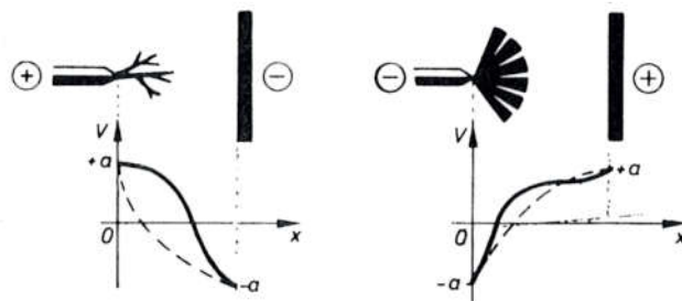
Sl. 404. Utjecaj polariteta na probojni napon
