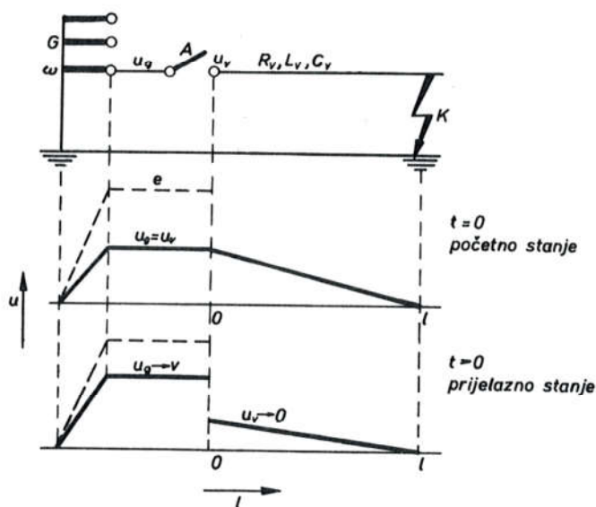
Sl. 6069. Bliski kratki spoj, shematski prikaz
