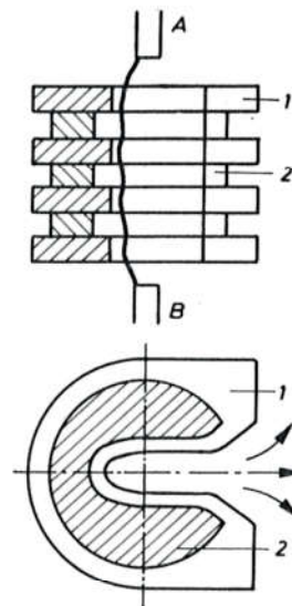
Sl. 728. Uljna deion-komora
