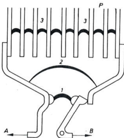
Sl. 762. Princip aparata s deion-rešetkom
