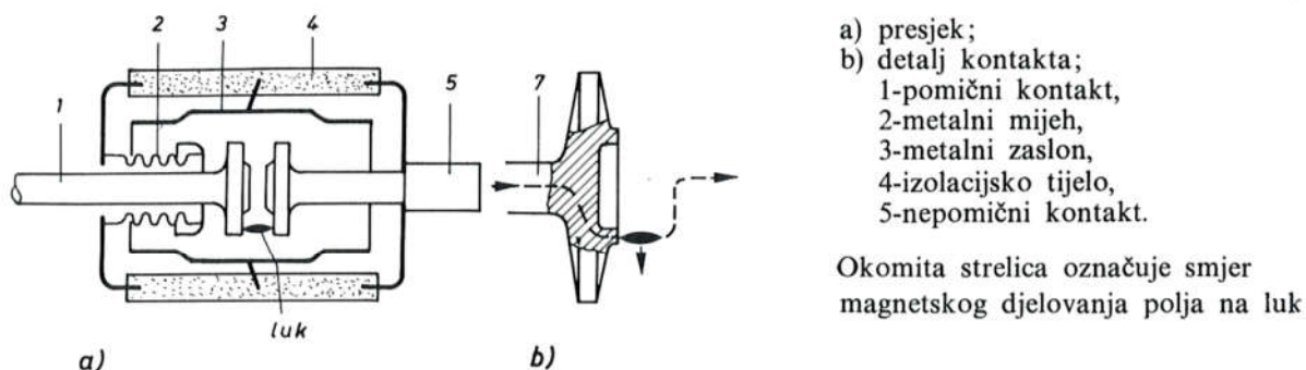
Sl. 764. Vakuumska lučna komora
