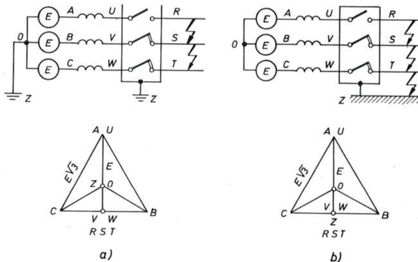
Sl. 766. Naponske prilike u polu koji prvi prekida:
