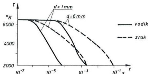
Sl. 709. Površinsko hlađenje rezidualnog stupca
