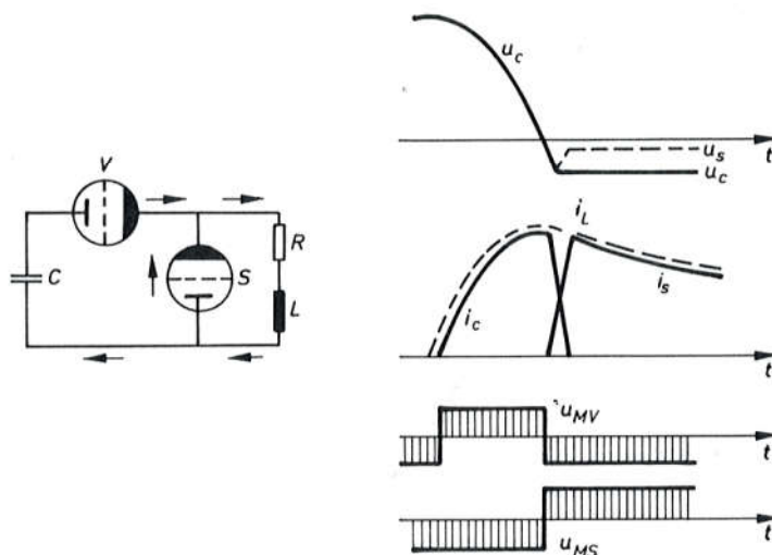
Sl. 706. Komutiranje jakih strujnih impulsa pomoću živinih ventila
