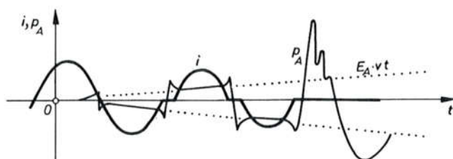
Sl. 6108. Oscilogram gašenja luka koji traje nekoliko poluperioda
