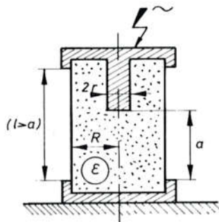
Sl. 416. Model potpornog izolatora s upuštenom gornjom elektrodom
