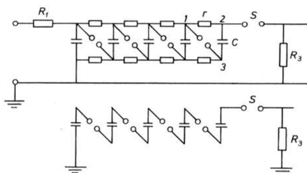
Sl. 409. Višestepeni udarni generator
