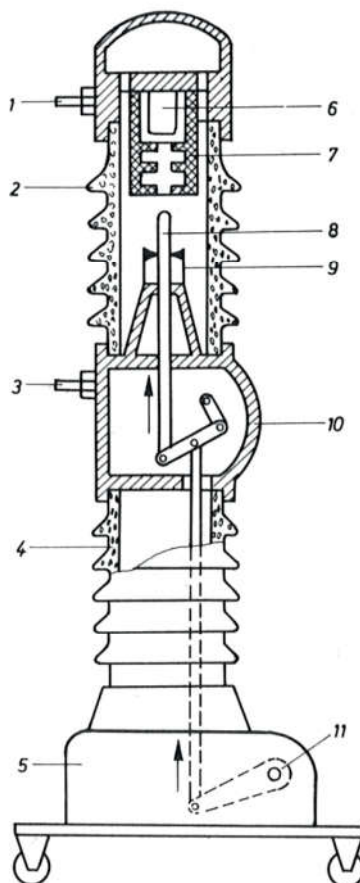
Sl. 724. Shematski prikaz malouljnog prekidača:
