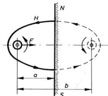
Sl. 503. Privlačne sile između vodiča i željezne stijene
