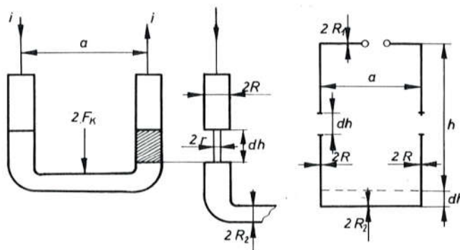
Sl. 516. Proračun odbojnih sila na kontaktnom mostu
