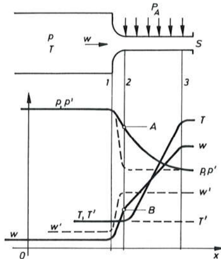
Sl. 737. Utjecaj topline luka na strujanje plina
