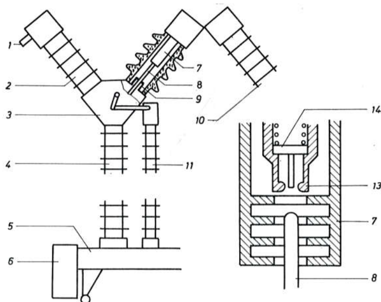
Sl. 730. Izvedba malouljnjog prekidača s komorama u obliku slova V
