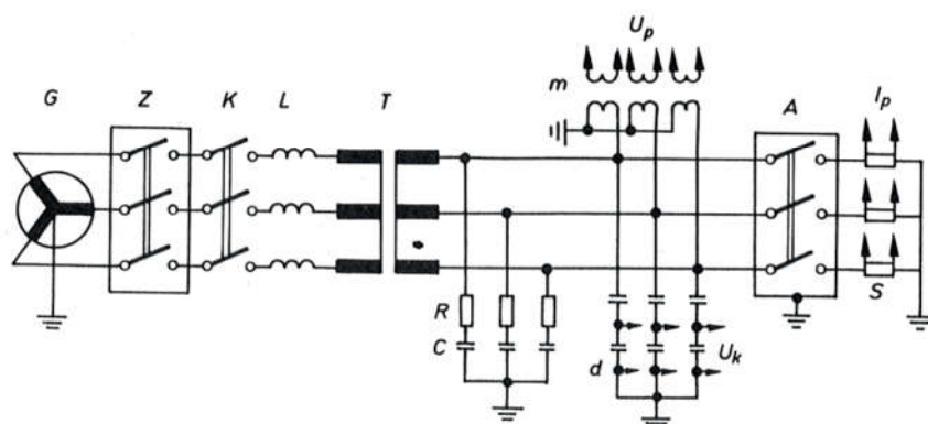
Sl. 765. Shema direktnog trofaznog ispitivanja prekidne moći:
