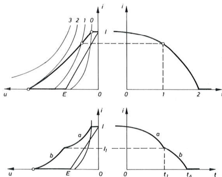
Sl. 6099. Gašenje luka promjenljive duljine u induktivnom krugu
