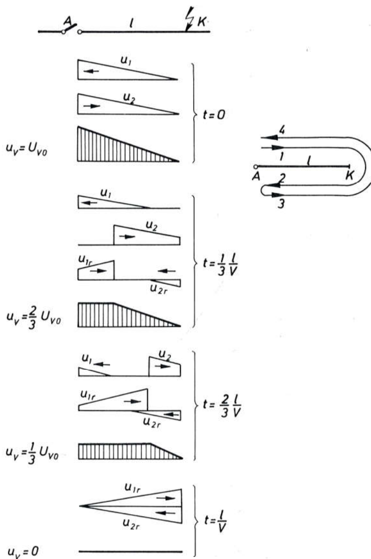
Sl. 6073. Putni valovi napona na dalekovodu
