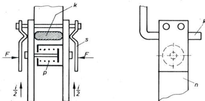
Sl. 511. Jačanje kontaktnog pritiska pomoću paralelnih noževa i elektromagnetskih steznika
