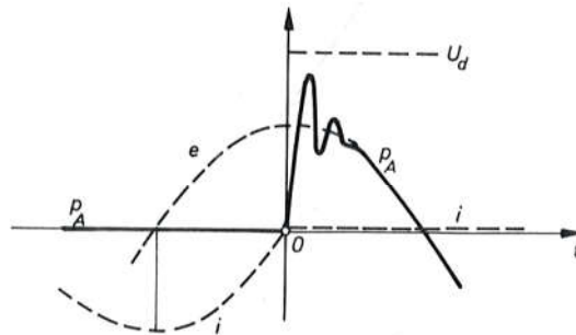
Sl. 6106. Dijagram prekidanja idealnog prekidača izmjenične struje
