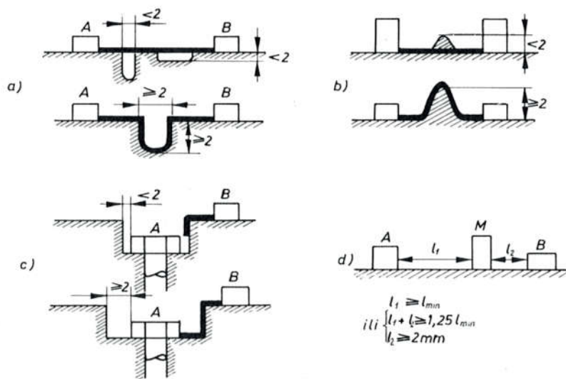
Sl. 426. Praktične smjernice za određivanje kliznih staza i izolacijskih razmaka
