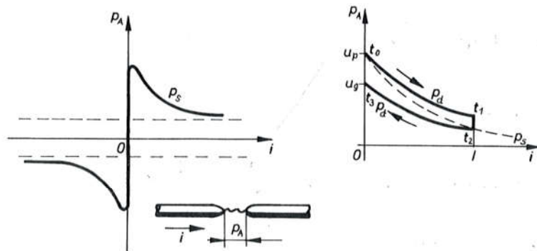
Sl. 6008. Statička i dinamička karakteristika luka
