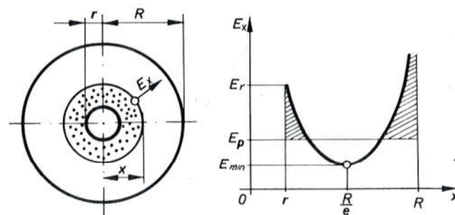
Sl. 402. Proces tinjanja među koaksijalnim elektrodama
