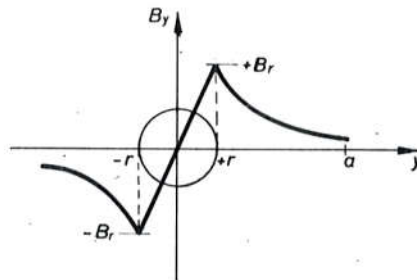
Sl. 506. Raspodjela indukcije u nožu
