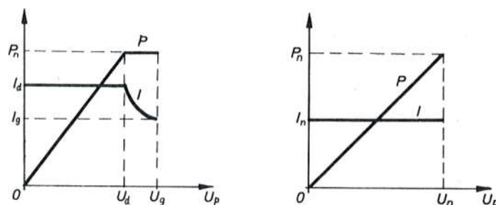
Sl. 6061. Prekidna moć kao funkcija povratnog napona
