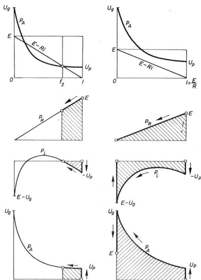
Sl. 6092. Varijacije padova napona u procesu neuspjelog i uspjelog gašenja luka
