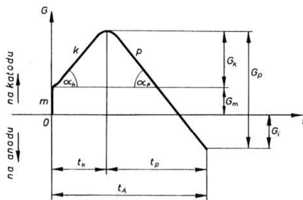
Sl. 214. Prijenos materijala za vrijeme isklapanja
