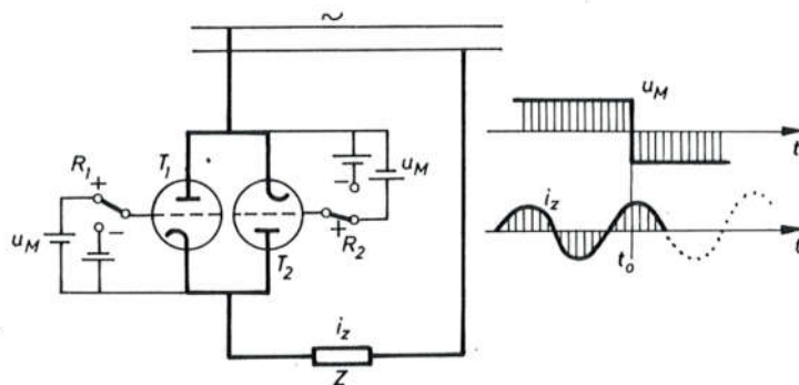
Sl. 705. Beskontaktno prekidanje pomoću tiratrona
