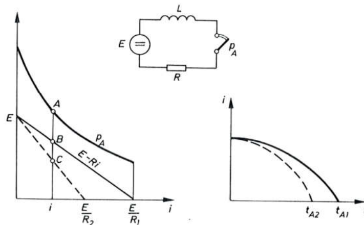
Sl. 6095. Utjecaj konstante L/R na trajanje luka t_A
