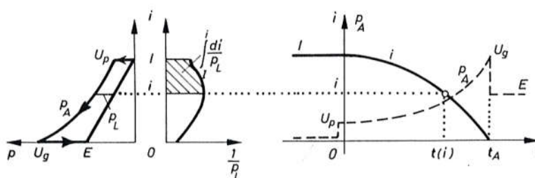
Sl. 6093. Grafičko određivanje krivulja i(t) i p_A(t)
