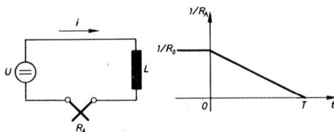
Sl. 6054. Promjena vodljivosti sklopke pri isklapanju
