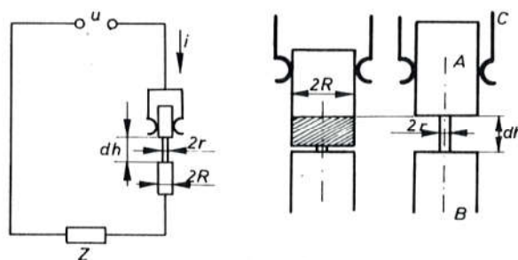
Sl. 512. Određivanje odbojnih sila među kontaktima s točkastim dodirom
