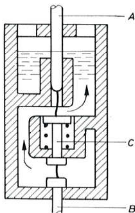
Sl. 725. Lučna komora s primarnim lukom
