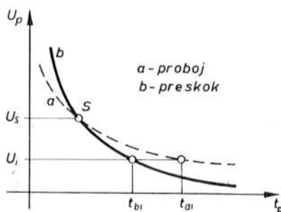
Sl. 415. Probojne i preskočne karakteristike za slučajeve a) i b) na slici 414.
