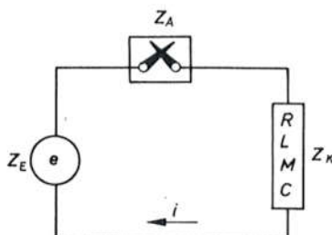
Sl. 6002. Primjer strujnoga kruga koji se sastoji od izvora energije, potrošača i sklopnog aparata energije, Z_A otpor sklopnog aparata, a Z_K rezultatni otpor preostalog dijela kruga, sastavljen bilo od kakve kombinacije omskih otpora R , samoinduktiviteta L , međuinuktiviteta M i kapaciteta C .
