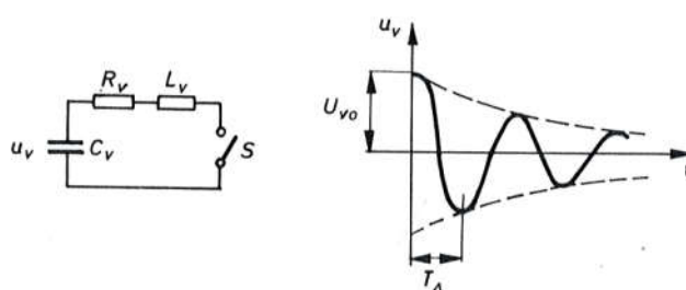
Sl. 6074. Pojednostavljena ekvivalentna shema i prigušeni sinusni titraji koji aproksimiraju pilasti napon
