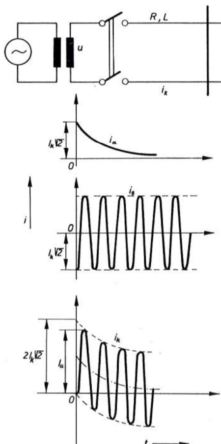
Sl. 6050. Struja kratkog spoja uz pretpostavku konstantne reaktancije izvora
