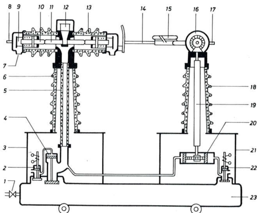
Sl. 743. Shematski presjek pneumatskog prekidača
