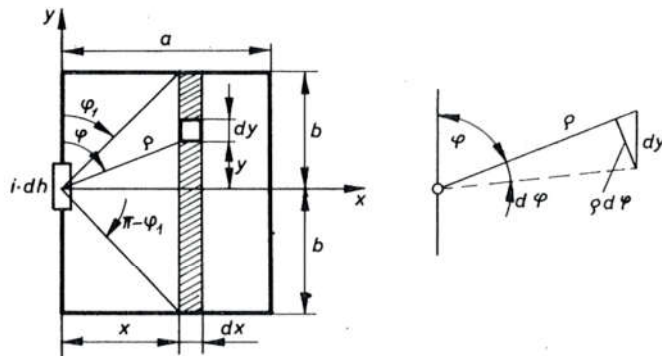
Sl. 515. Proračun koeficijenata K_1 i K_2 za pravokutnu strujnu petlju
