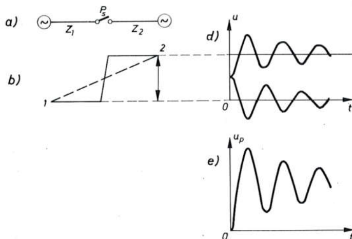
Sl. 6081. Promjena napona pri isklapanju dvaju sistema jednakih impedancija
