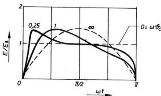
Sl. 6040. Gradijent luka sinusne struje po Cassieu
