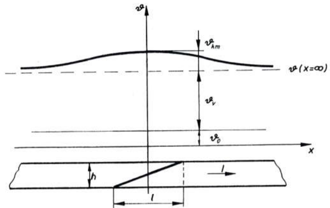
Sl. 305. Klinasti spoj vodiča
