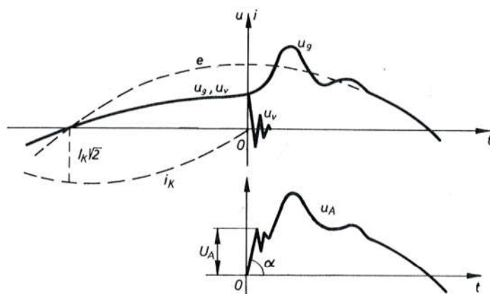
Sl. 6070. Povratni napon pri bliskom kratkom spoju
