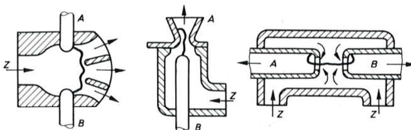
Sl. 734. Lučne komore pneumatskih prekidača
