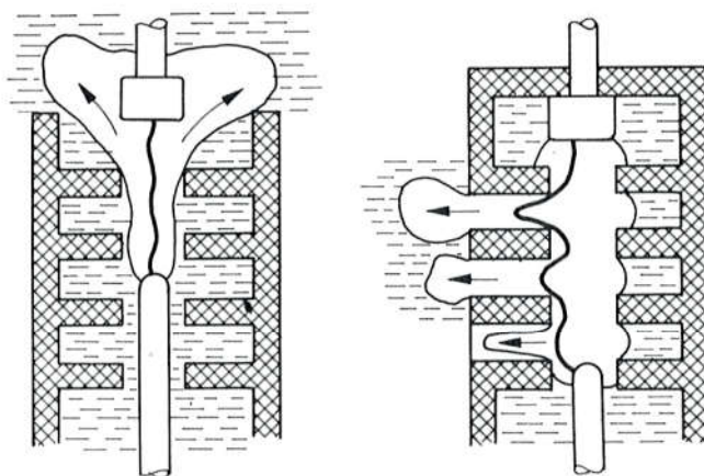
Sl. 723. Lučne komore malouljnih prekidača
