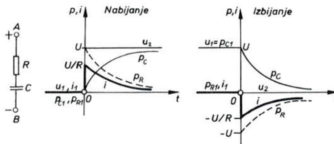
Sl. 6045. Nabijanje i izbijanje kondenzatora
