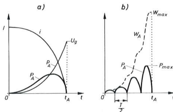
Sl. 6101. Snaga i energija luka: a) istosmjerna struja, b) izmjenična
