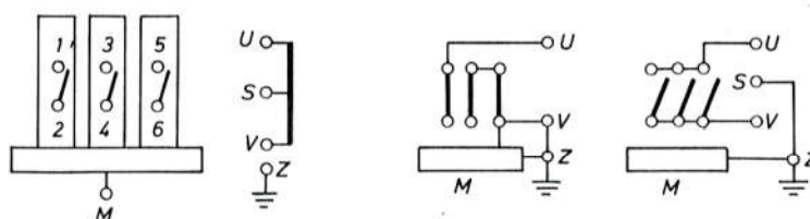
Sl. 420. Sheme ispitnih spojeva
