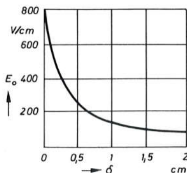
Sl. 758. Utjecaj širine raspora na luk koji miruje
