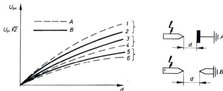
Sl. 410. Amplitude probojnih napona u zraku atmosferskog pritiska
