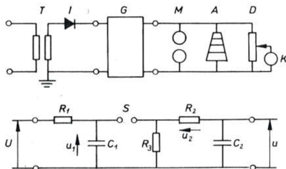
Sl. 407. Ispitivanje udarnim naponom
