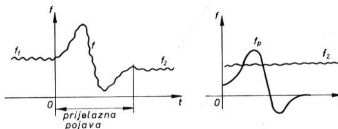
Sl. 6001. Dijagram prijelazne pojave i njezinih komponenata
