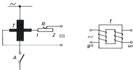
Sl. 704. Aparati na principu transduktora
