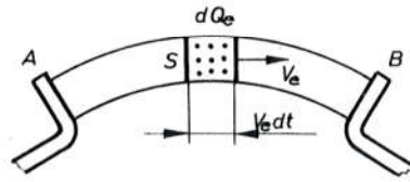
Sl. 6023. Određivanje specifičnog otpora luka
