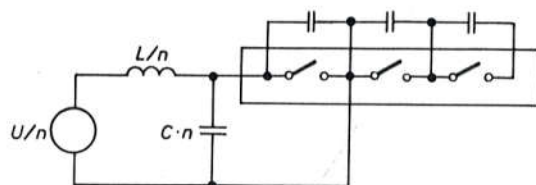
Sl. 768. Ispitivanje po elementima. Prekidač ima tri prekidna elementa po fazi
