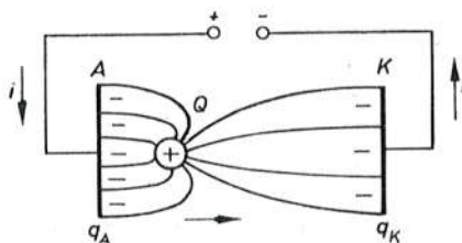
Sl. 6012. Struja nesamostalnog izbijanja
