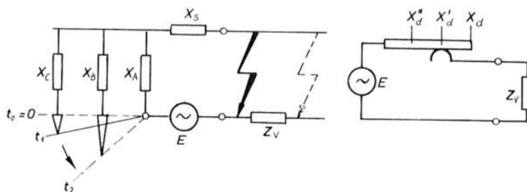
Sl. 6052. Shematski prikaz reaktancija sinhronog stroja u kratkom spoju
