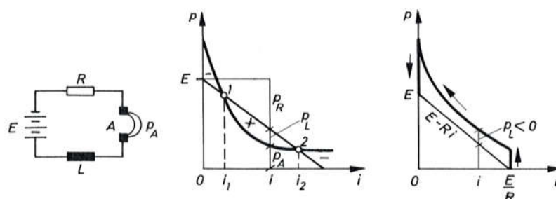
Sl. 6091. Kriterij nestabilnosti luka
