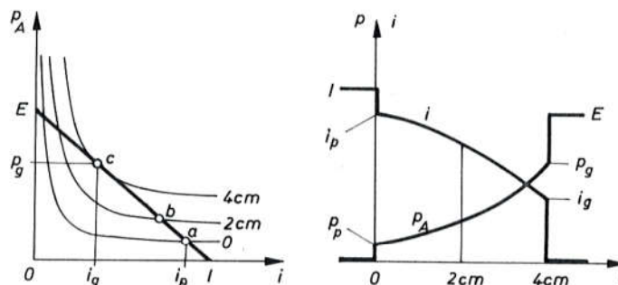
Sl. 6096. Gašenje luka u omskom krugu istosmjerne struje
