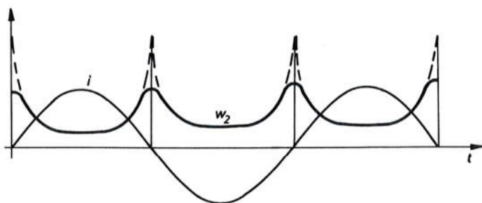
Sl. 740. Utjecaj struje na brzinu komprimiranog zraka
