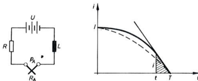
Sl. 6056. Struja prekidanja u krugu R-L
