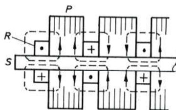
Sl. 763. Stvaranje radijalnog magnetskog polja za rotaciju luka
