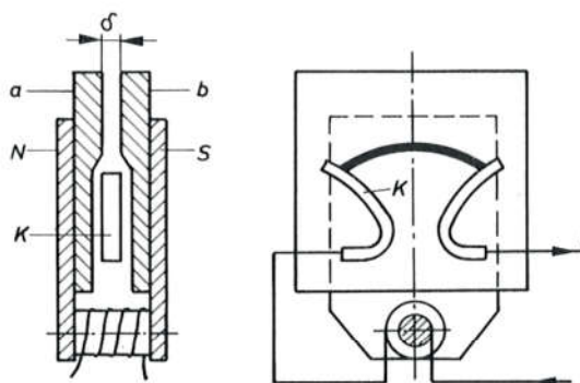
Sl. 757. Komora aparata s uskim rasporima
