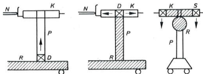
Sl. 741. Napajanje lučne komore komprimiranim zrakom: osjenčano – pod stalnim pritiskom, – ventili
