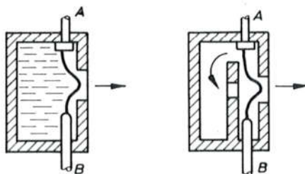
Sl. 716. Princip lučnih komora sa zavisnom karakteristikom
