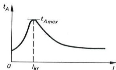
Sl. 717. Trajanje luka i kritična struja
