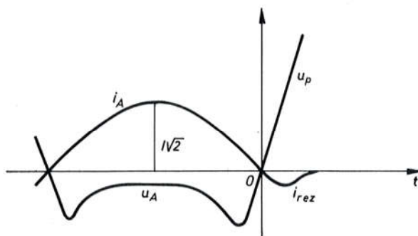
Sl. 713. Gašenje luka uz linearni porast povratnog napona
