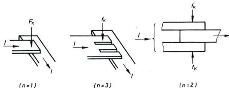
Sl. 313. Povećanje termičke otpornosti kontakata
