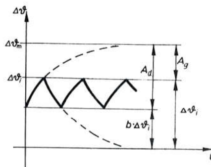
Sl. 309. Stacionarno stanje intermitiranog pogona
