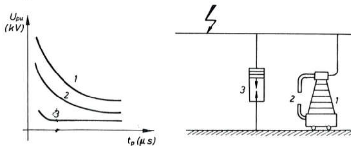
Sl. 418. Koordinacije izolacije:
