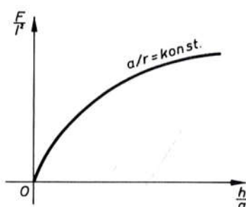
Sl. 508. Sila na nož rastavljača kao funkcija geometrijskih odnosa
