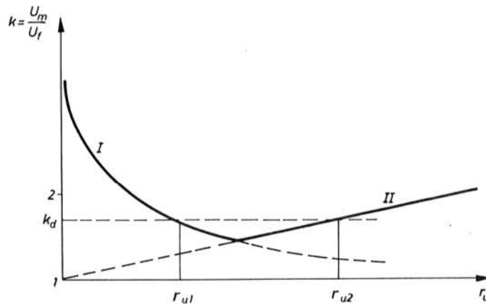
Sl. 6089. Ovisnost najvećeg prenapona o veličini uklopnog otpora r_u
