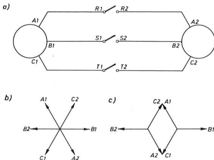
Sl. 6079. Isklapanje u opoziciji faza
