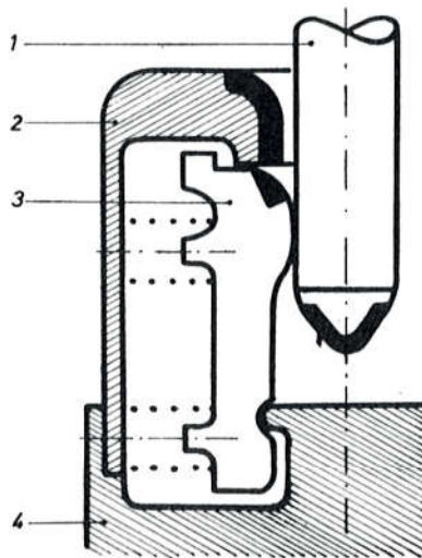
Sl. 213. Primjena sinterovanih materijala na kontaktima prekidača
