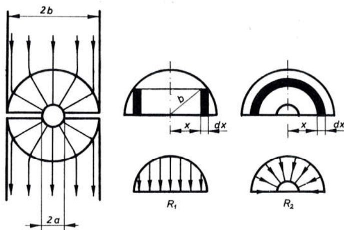
Sl. 203. Proračun provlačnog otpora
