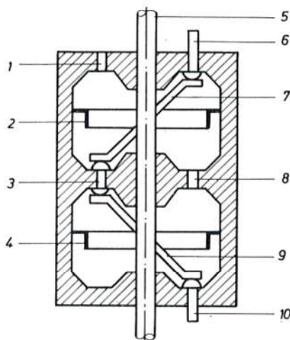
Sl. 729. Shema komore rotacionog prekidača s višestrukim prekidom
