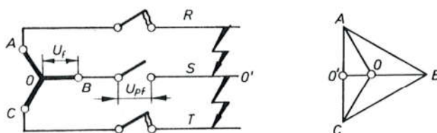
Sl. 6059. Povišenje povratnog napona na polu koji prvi prekida struju
