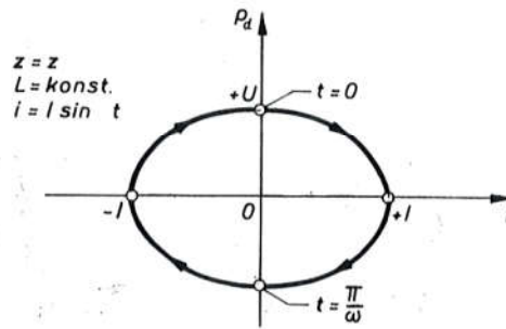
Sl. 6007. Dinamička karakteristika prigušnice
