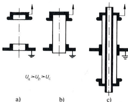
Sl. 414. Utjecaj krutog izolatora na preskočni napon
