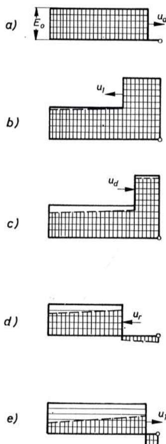
Sl. 6086. Naponski putni val od uklapanja neopterećenog nenabijenog voda
