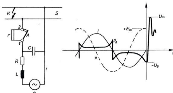
Sl. 6057. Shema i oscilogram prekidanja kratkog spoja u induktivnom krugu izmjenične struje
