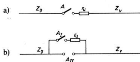
Sl. 6088. Uklapanje voda pomoću uklopnog otpora
