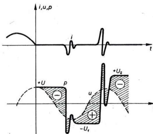
Sl. 6063. Prenaponi izazvani ponovnim paljenjem luka
