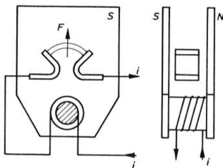
Sl. 6104. Produljivanje i gašenje luka pomoću magnetskog polja
