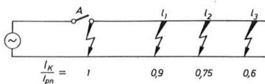
Sl. 6077. Ispitivanje prekidne moći pri bliskom kratkom spoju
