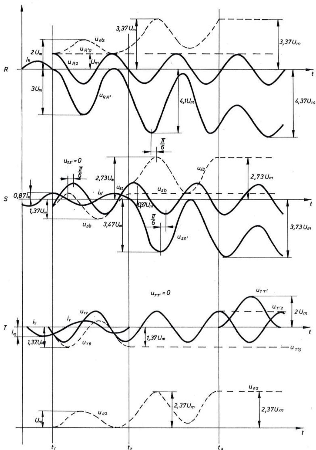
Sl. 6067. Uzastopno isklapanje jednog pola za drugu sklopke s priključenim neopterećenim kabelom
