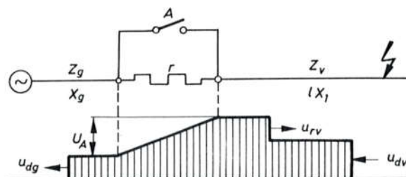
Sl. 6078. Ograničenje amplitude pilastog napona pomoću paralelnih otpora
