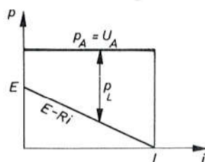
Sl. 6094. Proračun trajanja luka uz p_A = \text{konst}
