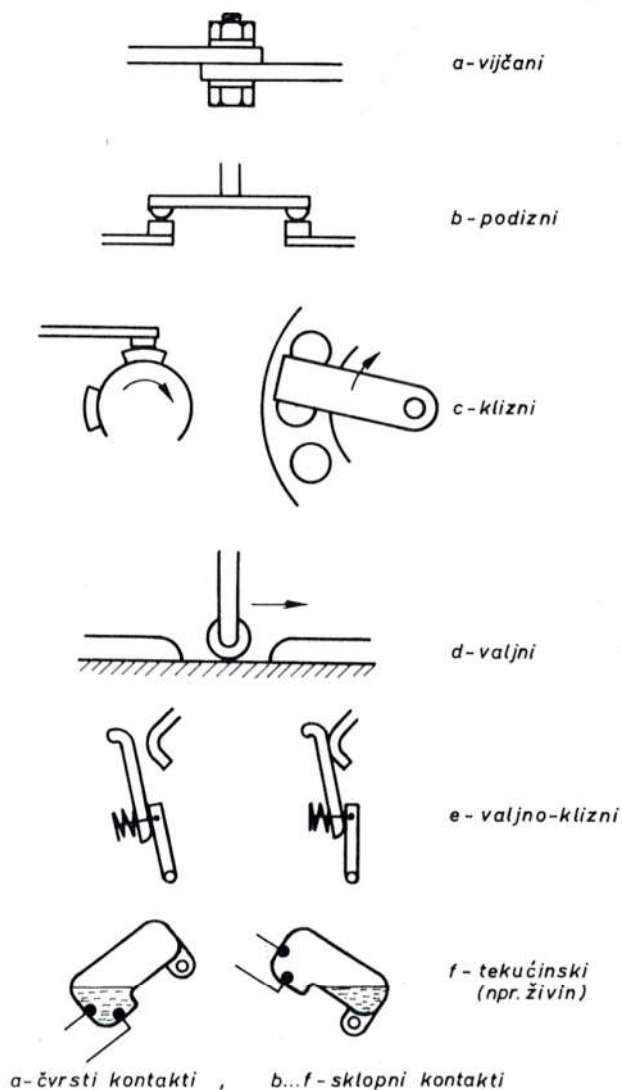
Sl. 315. Izvedbe kontakta s obzirom na način gibanja
