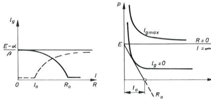
Sl. 6097. Duljina luka u trenutku gašenja
