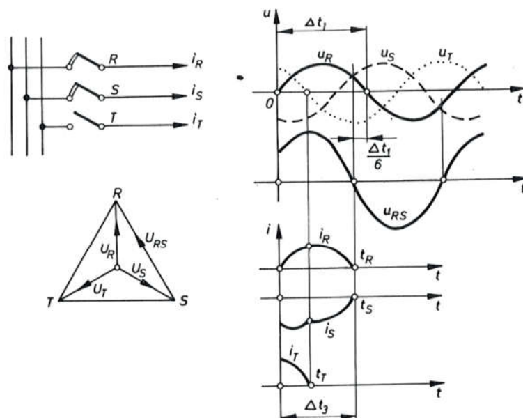
Sl. 719. Određivanje veličine \Delta t za trofaznu struju
