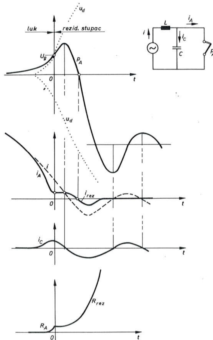
Sl. 6109. Rezidualna struja u oscilogramu prekidanja
