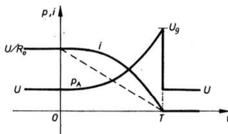
Sl. 6055. Utjecaj otpora sklopke na prijelazne pojave struje i napona
