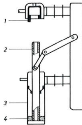
Sl. 748. Autopneumatska rastavna sklopka
