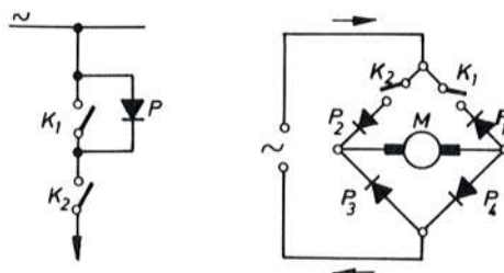
Sl. 703. Prekidanje bez luka primjenom poluvodičkih ispravljača
