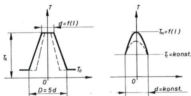
Sl. 6037. Modeli raspodjele temperature u luku
