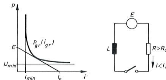
Sl. 6098. Prekidanje bez pojave luka
