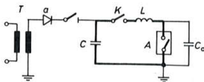
Sl. 769. Ispitni titrajni krug po Gorevu:
