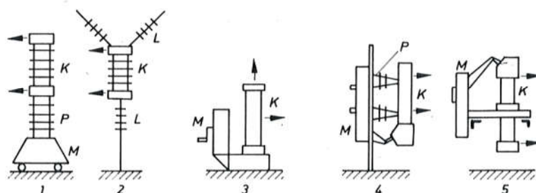
Sl. 732. Montažni oblici malouljnih prekidača
