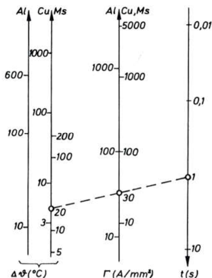
Sl. 311. Nomogram zagrijavanja vodiča u kratkom spoju. Primjer očitavanja za mjed (Ms):
