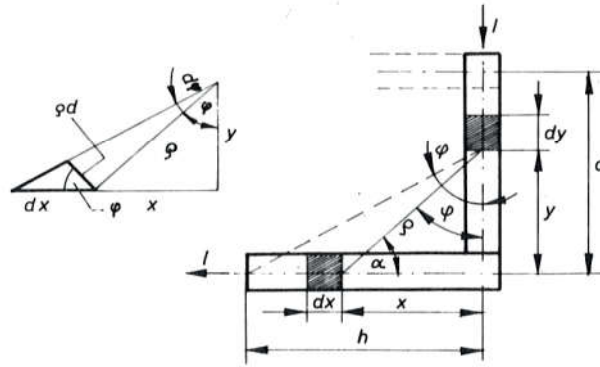
Sl. 505. Proračun »vanjske« indukcije
