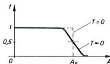
Sl. 6028. Funkcija Fermi-Diracove razdiobe
