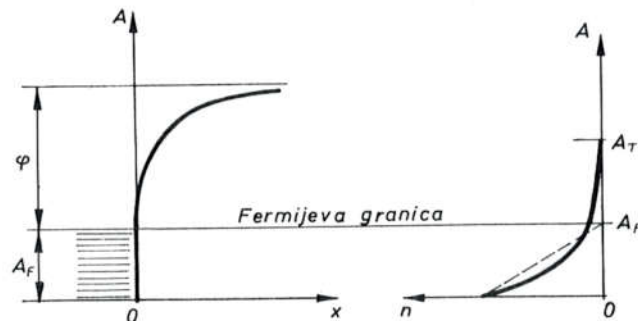
Sl. 6027. Elektronsko korito i Fermijeva granica
