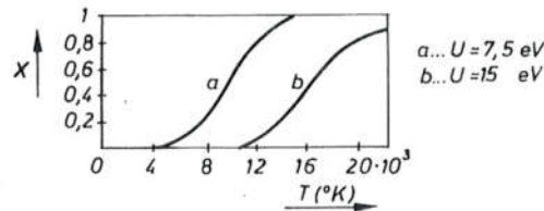
Sl. 6016. Stupanj termičke ionizacije za metalne pare (a) i plinove (b) uz tlak p = 1 \text{ kp/cm}^2
