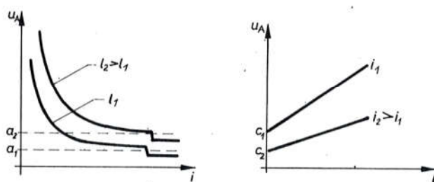
Sl. 6033. Statičke karakteristike luka uz konstantnu duljinu i konstantnu struju
