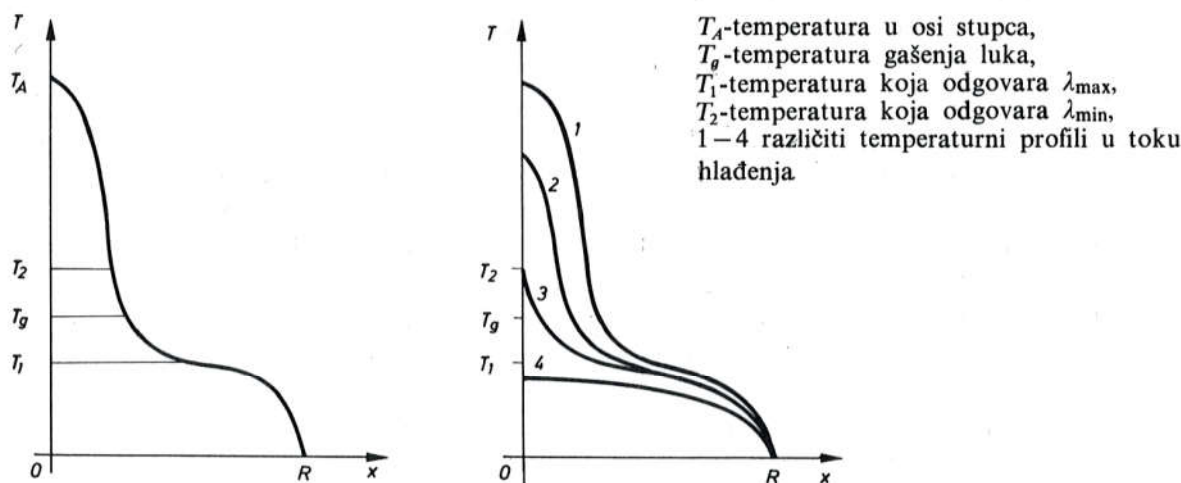
Sl. 750. Temperaturni profil luka u \text{SF}_6 unutar hladne cijevi polumjera R
