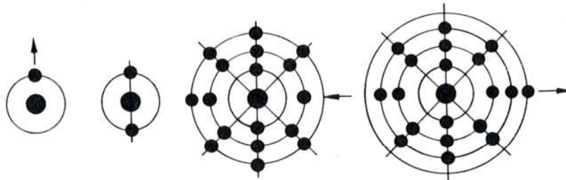
Sl. 401. Ilustracija električnih svojstava pomoću Bohrovih atomskih modela
