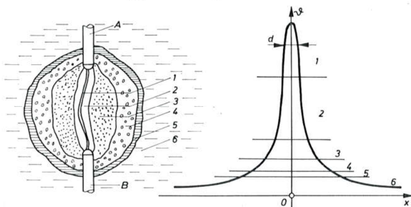
Sl. 721. Sastav i temperatura plinskog mjehura
