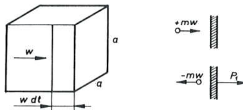
Sl. 6017. Kinetička predodžba tlaka u plinovima
