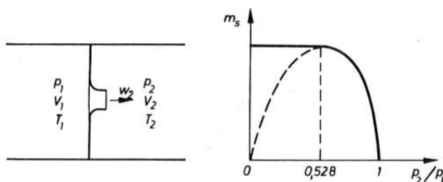
Sl. 736. Adijabatsko strujanje plina
