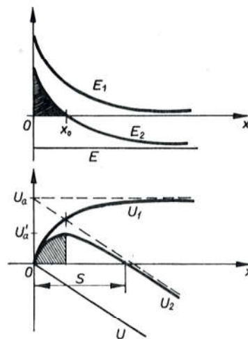
Sl. 6025. Utjecaj vanjskog polja na potencijalnu barijeru
