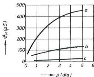
Sl. 6043. Zavisnost vremenske konstante od vrste plina i njegova tlaka:
