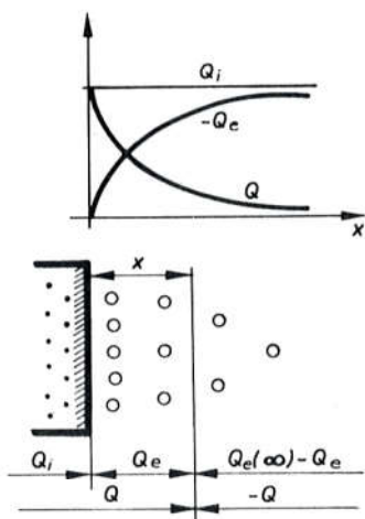
Sl. 6024. Raspodjela naboja na prijelazu metal – plin
