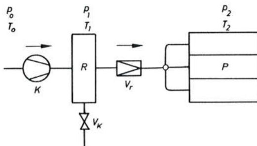
Sl. 747. Utjecaj kompresije i redukcije tlaka na vlažnost zraka
