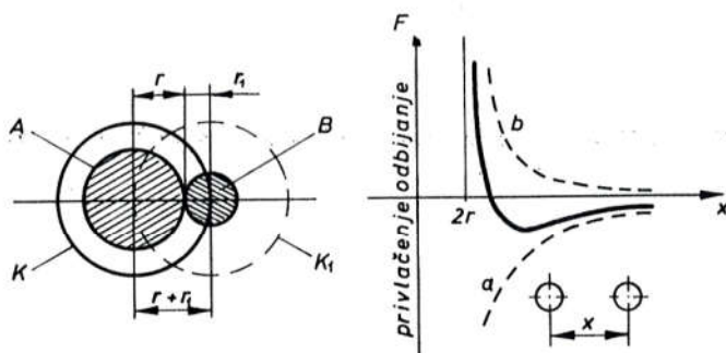
Sl. 6019. Udarni presjek čestica i međumolekularne sile
