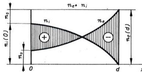
Sl. 6014. Prostorna raspodjela naboja
