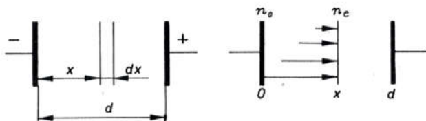
Sl. 6013. Stvaranje lavine udarnom ionizacijom
