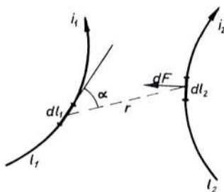
Sl. 501. Primjena Biot-Savartova zakona
