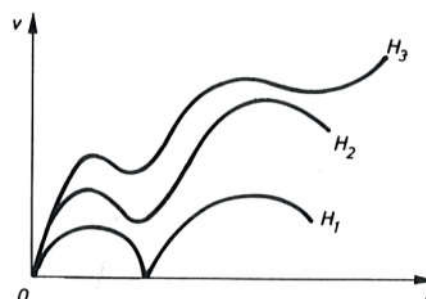
Sl. 759. Brzina kretanja luka u uskom rasporu
