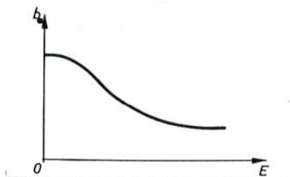
Sl. 6021. Pokretljivost elektrona kao funkcija jakosti polja
