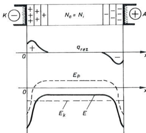
Sl. 6022. Resultantna gustoća naboja i električno polje u stupcu luka
