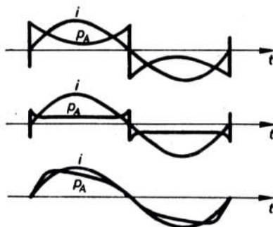
Sl. 6038. Utjecaj hlađenja na gradijent luka
