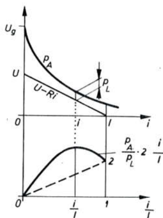
Sl. 6102. Proračun energije luka u krugu istosmjerne struje
