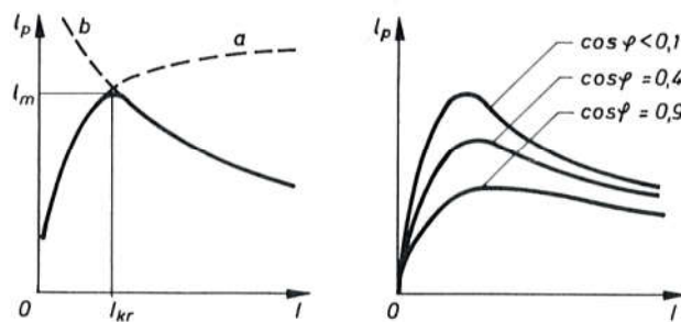
Sl. 711. Probajni razmak kao funkcija struje koja je prije toga tekla u luku
