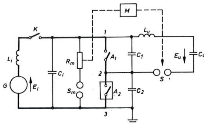
Sl. 776. Siemensov »komponentni spoj II«: G-generator, K-kratkospojnik, S_m -mjerno iskrište, A_1 -pomoćni prekidač, A_2 -ispitni prekidač, M-upravljački uređaj iskrišta S za uključivanje visokonaponskog kruga, C_u -nabijena kondenzatorska baterija kao izvor visokog napona
