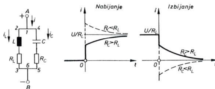
Sl. 6047. Paralelni spoj kondenzatora i prigušnice
