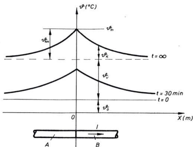
Sl. 302. Zagrijavanje kontakta prolazom struje
