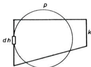
Sl. 514. Određivanje magnetskog toka koji element vodiča šalje kroz vlastitu petlju K
