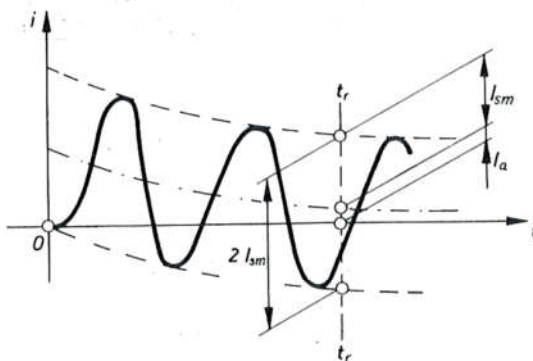
Sl. 6060. Određivanje prekidne struje iz oscilograma
