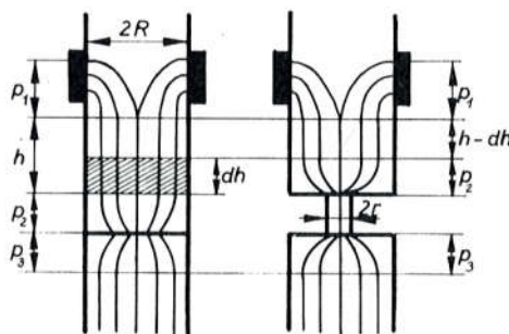
Sl. 513. Promjena strujnica zbog virtualnog pomaka
