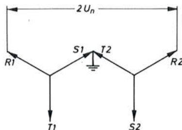
Sl. 6083. Naponi dvaju sistema koji su fazno pomaknuti nakon isklapanja istovremenih zemnih spojeva u oba sistema
