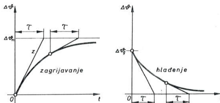
Sl. 307. Zagrijavanje i hlađenje u trajnom pogonu
