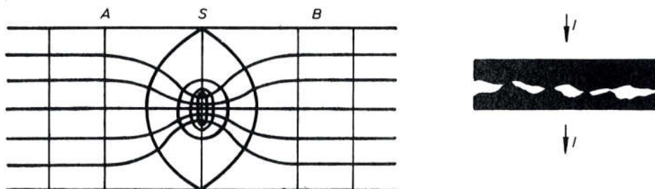
Sl. 202. Koncentracija strujnica i mikrostruktura dodirne plohe
