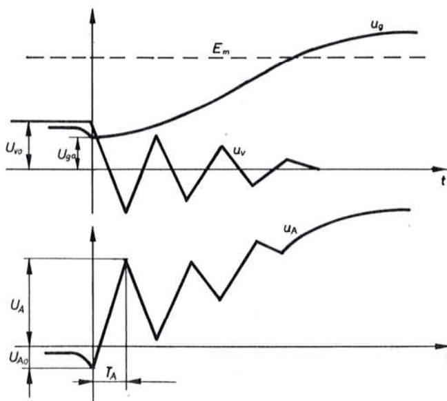
Sl. 6071. Pilasti oblik titranja napona neposredno nakon gašenja luka
