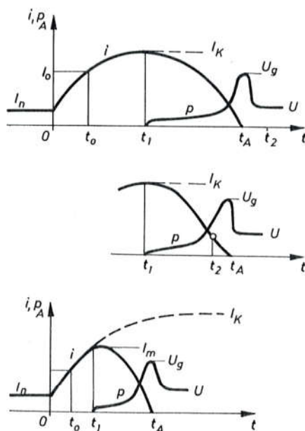
Sl. 6105. Dijagrami prekidanja kratkog spoja pomoću običnih i ultrabrzih prekidača za istosmjernu struju
