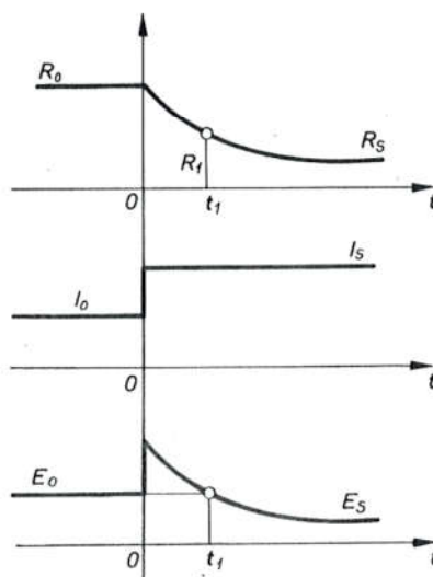
Sl. 6042. Eksperimentalno određivanje vremenske konstante luka
