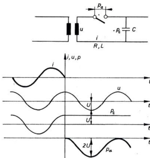
Sl. 6062. Shema isklapanja neopterećenog dalekovoda i pojednostavljena slika prenapona
