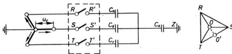
Sl. 6065. Nadoknadna shema strujnog kruga neopterećenog kabela
