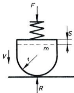
Sl. 210. Sudar kontakta pri uklopu
