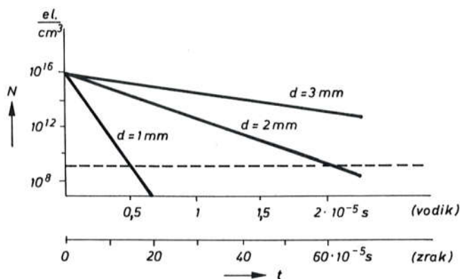
Sl. 708. Deionizacija rezidualnog stupca difuzijom
