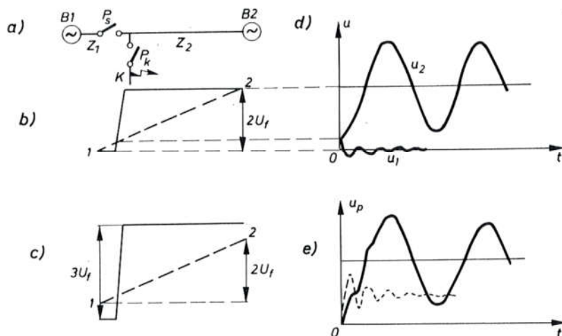
Sl. 6080. Promjena napona pri isklapanju dvaju sistema raznih impedancija
