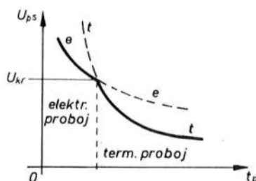
Sl. 417. Ovisnost vremena proboja o statičkom probojnom naponu
