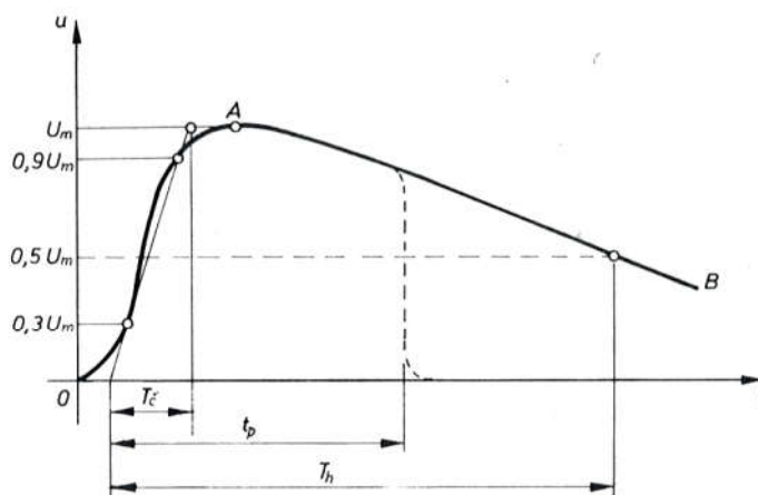
Sl. 405. Standardni oblik vala udarnog napona
