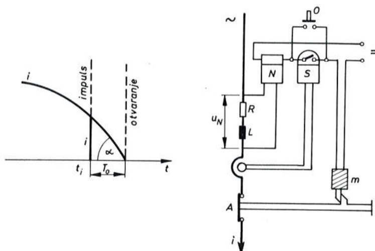
Sl. 702. Princip djelovanja sinhronog prekidača
