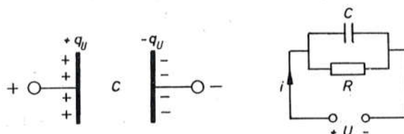
Sl. 6011. Shema kruga s plinovitim medijem
