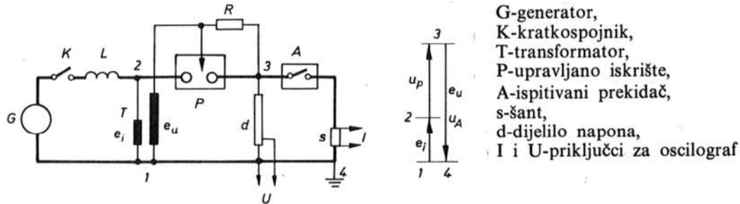
Sl. 772. Sintetski krug tvrtke »Merlin &amp; Gerin«
