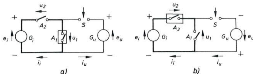
Sl. 770. Načelna shema sintetskog ispitivanja. Naponski izvor G_u priključen paralelno: a) ispitnom prekidaču; b) pomoćnom prekidaču;
