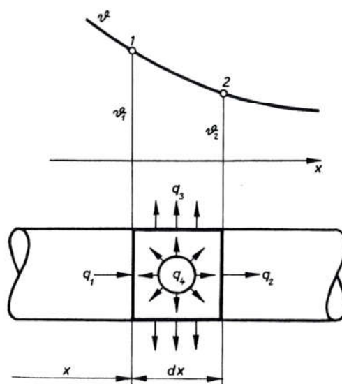
Sl. 303. Kretanje topline u elementu vodiča
