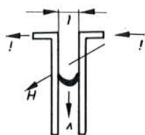
Sl. 756. Gašenje luka među paralelnim rogovima
