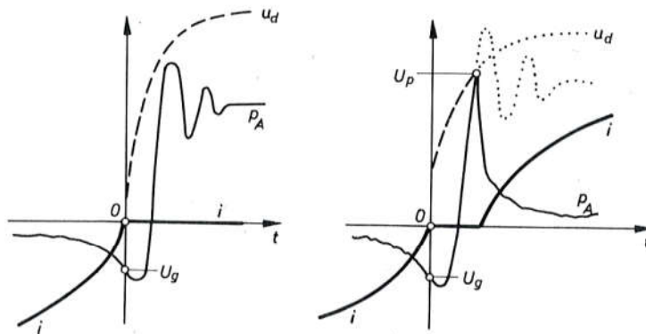
Sl. 6107. Dijagrami prekidanja izmjenične struje
