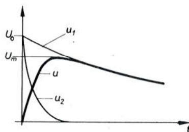
Sl. 408. Udarni val u = u_1 - u_2
