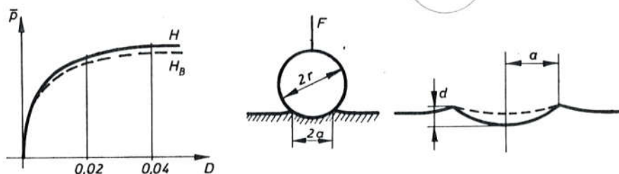
Sl. 205. Određivanje tvrdoće kontaktnog materijala
