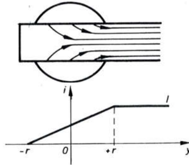
Sl. 507. Približna razdioba struje u nožu
