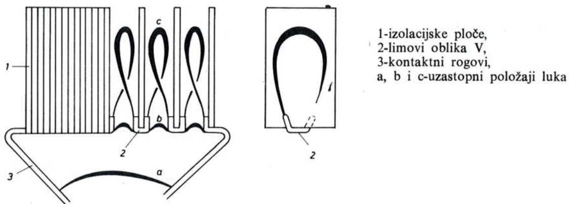
Sl. 761. Aparat sa spiralnim lukom (»solenarc«)
