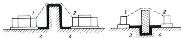
Sl. 424. Izolacijski razmaci i klizne staze
