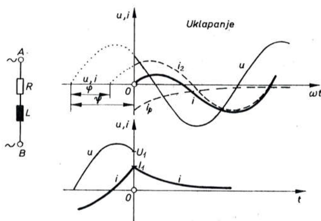
Sl. 6049. Induktivni krug izmjenične struje
