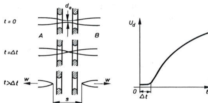
Sl. 735. Uspostavljanje električke čvrstoće u pneumatskoj komori
