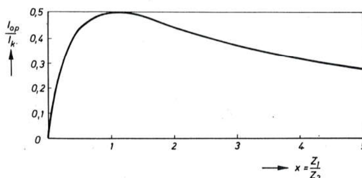
Sl. 6082. Omjer prekidnih struja pri opoziciji faza i kratkom spoju u ovisnosti o omjeru impedancija
