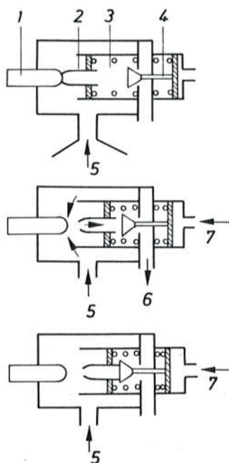
Sl. 742. Lučna komora pod stalnim pritiskom
