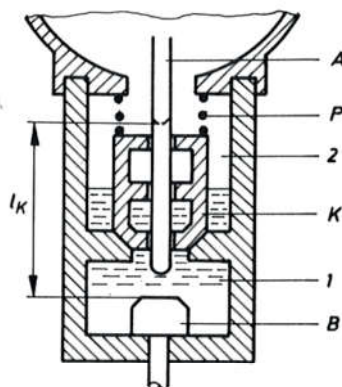
Sl. 733. Elastična komora hidromatskog prekidača
