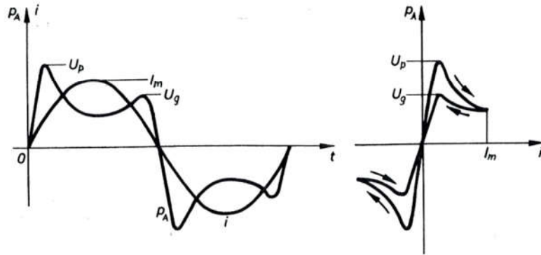
Sl. 6009. Dinamička karakteristika luka izmjenične struje
