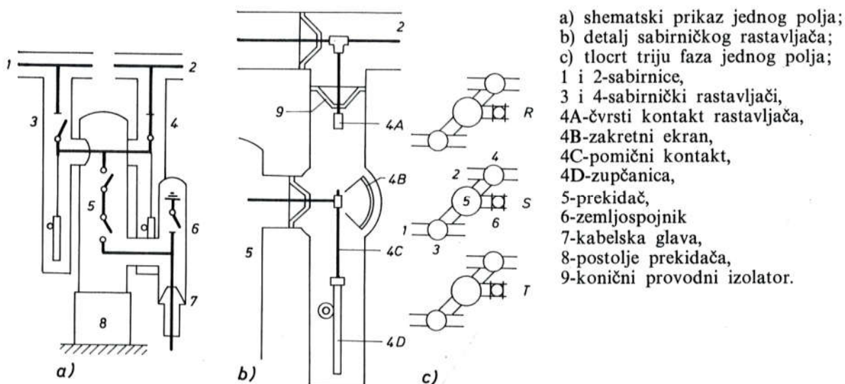
Sl. 755. Oklopno postrojenje izolirano plinom \text{SF}_6
