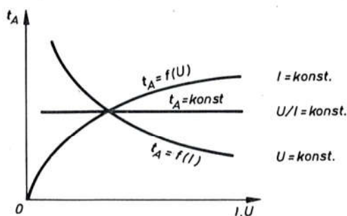
Sl. 720. Trajanje luka u prekidačima sa zavisnom karakteristikom kao funkcija struje i napona
