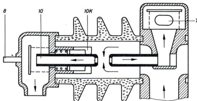
Sl. 744. Lučna komora pneumatskog prekidača u trenutku gašenja
