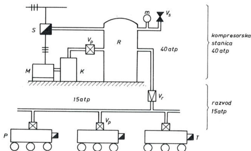
Sl. 745. Shema instalacije komprimiranog zraka:
