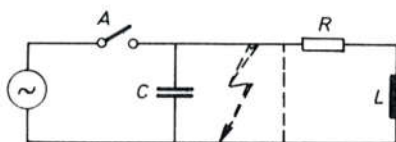
Sl. 6090. Shematski prikaz evolutivnog kvara
