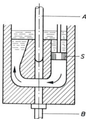
Sl. 727. Impulsna komora s mehaničkim potiskivanjem ulja
