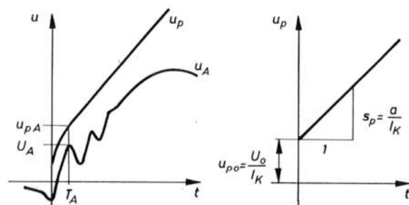
Sl. 6075. Vremenski dijagrami povratnih i probojnih napona
