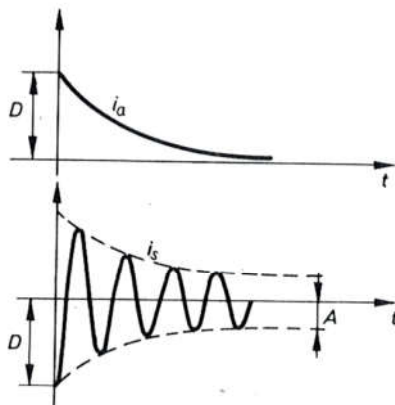
Sl. 6051. Aperiodska i simetrična komponenta struje kratkog spoja
