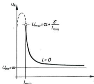
Sl. 6034. Granična karakteristika luka
