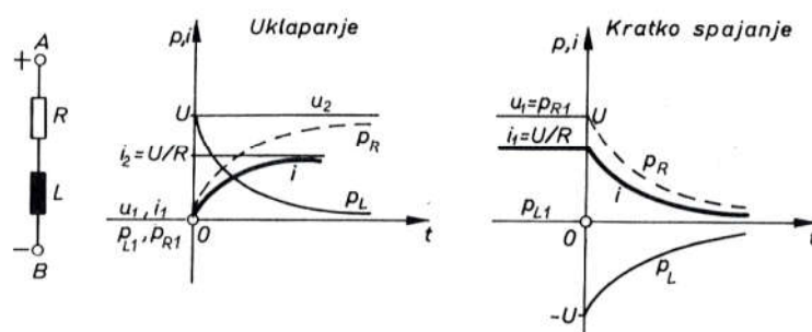
Sl. 6046. Uklapanje i kratko spajanje prigušnice
