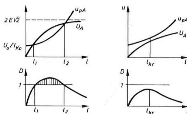
Sl. 6076. Faktor naprežanja, opasna zona i kritična udaljenost
