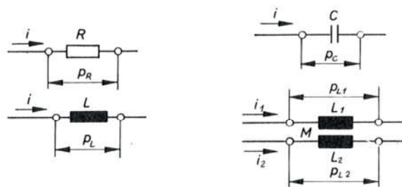
Sl. 6003. Pad napona na osnovnim tipovima impedancija
