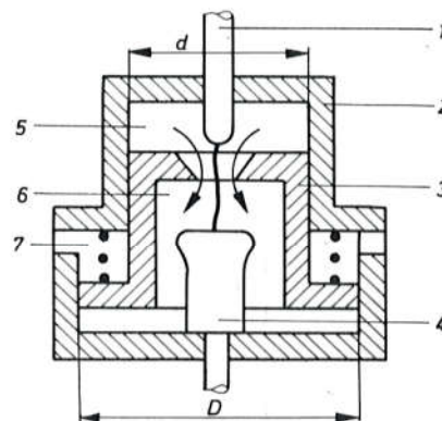
Sl. 726. Komora s diferencijalnim klipom
