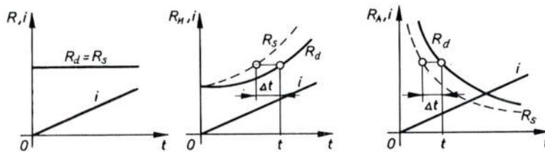
Sl. 6006. Statičke i dinamičke karakteristike R(t)
