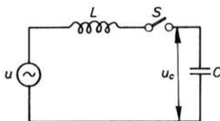
Sl. 6068. Jednopolna shema kruga s aparatom za uklapanje kondenzatora
