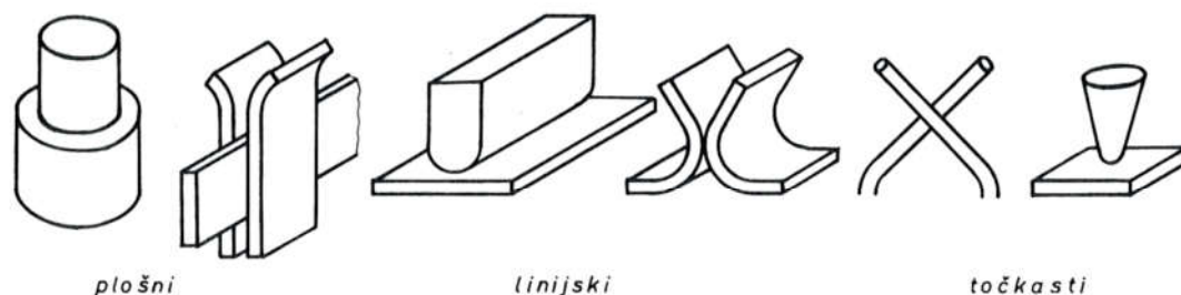
Sl. 316. Izvedbe kontakta s obzirom na oblik dodirne plohe
