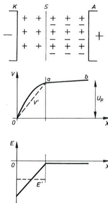
Sl. 714. Rezidualni stupac kratkog luka
