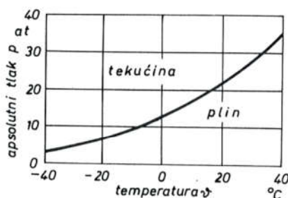
Sl. 752. Krivulja ravnoteže plin-tekućina za SF_6
