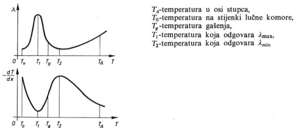
Sl. 749. Ovisnost toplinske vodljivosti \lambda i gradijenta temperature dT/dx lučnog stupca u \text{SF}_6 o temperaturi
