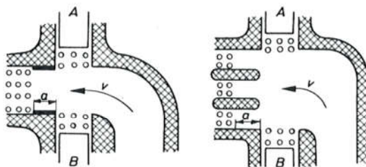
Sl. 712. Gašenje luka prema teoriji pomaka
