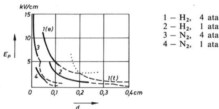
Sl. 710. Gradijent ponovnog paljenja u zavisnosti od promjera luka
