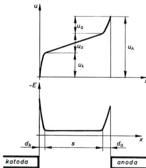
Sl. 6026. Prostorna razdioba napona i gradijenta u luku
