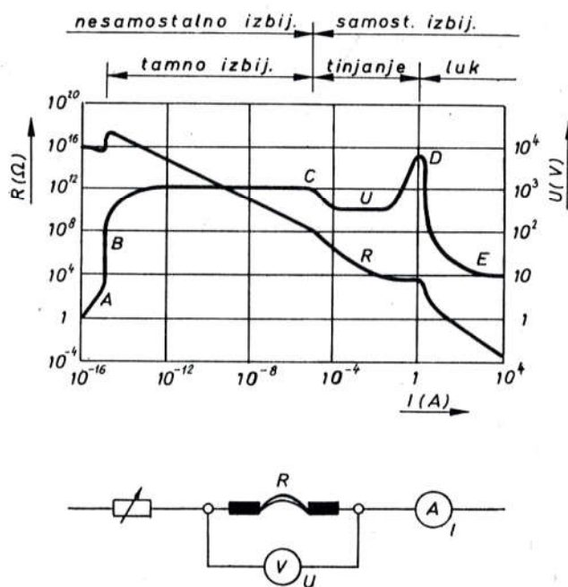
Sl. 6010. Karakteristike izbijanja u plinovima
