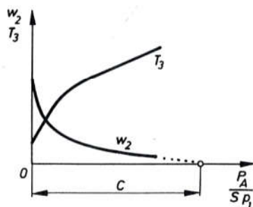
Sl. 739. Termodinamičko prigušivanje u sapnici pneumatskog prekidača
