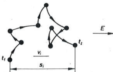
Sl. 6020. Kretanje iona u električnom polju
