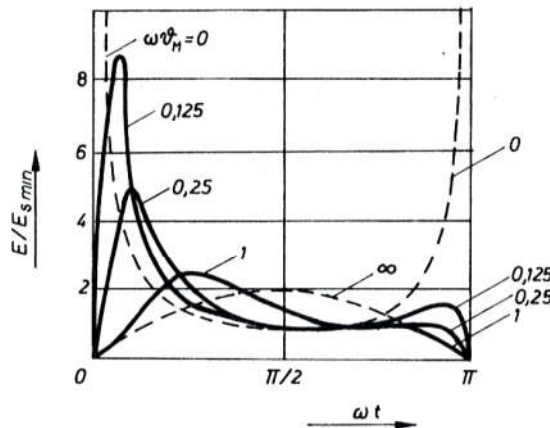
Sl. 6041. Gradijent luka sinusne struje po Mayru
