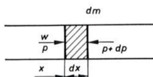
Sl. 738. Ilustracija zakona impulsa i energije
