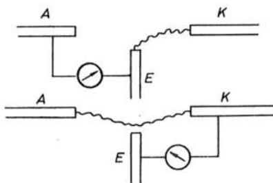
Sl. 6030. Flemingov pokus
