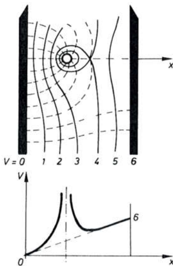
Sl. 403. Deformacija homogenog električnog polja točkastim prostornim nabojem
