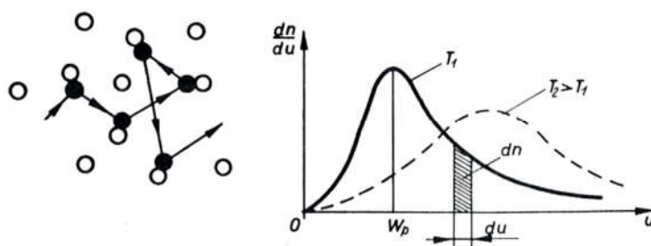
Sl. 6018. Maxwelllova raspodjela brzina
