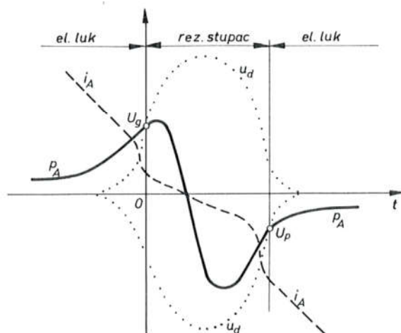
Sl. 6110. Ponovno paljenje luka izazvano termičkim procesima u rezidualnom stupcu
