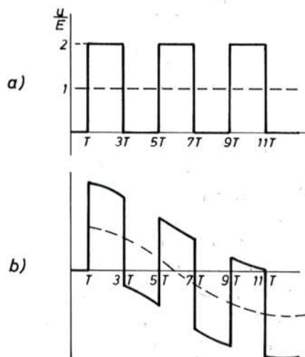
Sl. 6087. Vremenska promjena napona na otvorenom kraju voda
