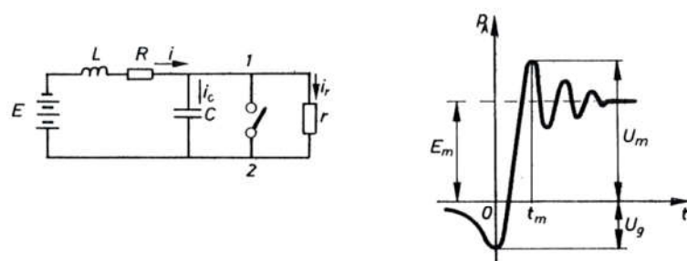
Sl. 6058. Ekvivalentna shema i povratni napon
