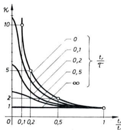
Sl. 310. Preopteretivost aparata u intermitiranom pogonu
