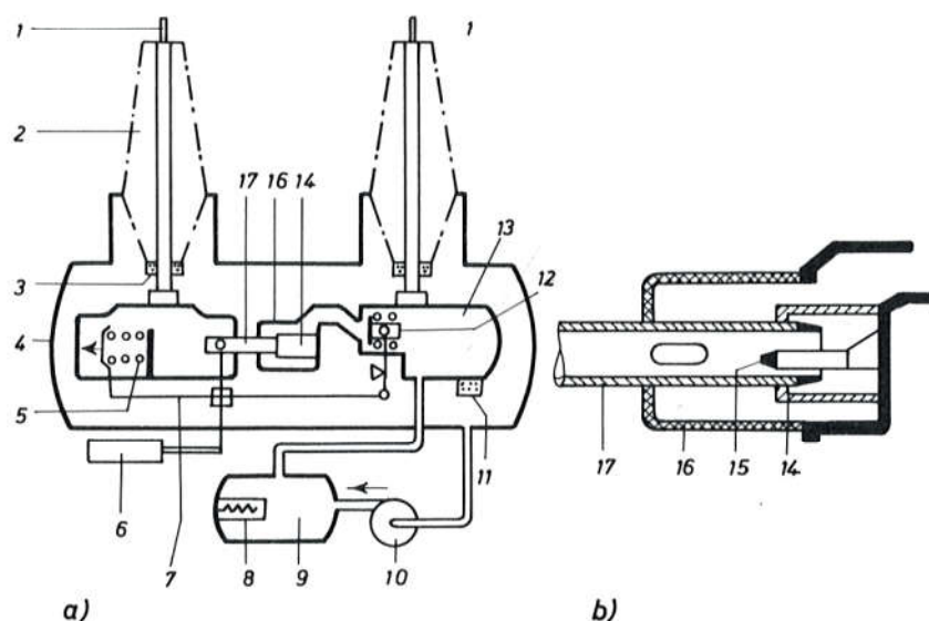
Sl. 753. Dvotlačni prekidač sa sumpornim heksafluoridom:
