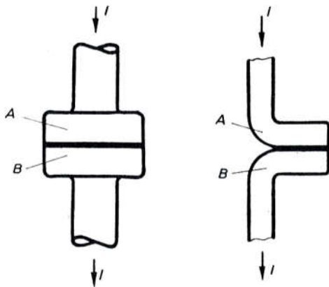
Sl. 304. Lokalno povećanje presjeka na kontaktima
