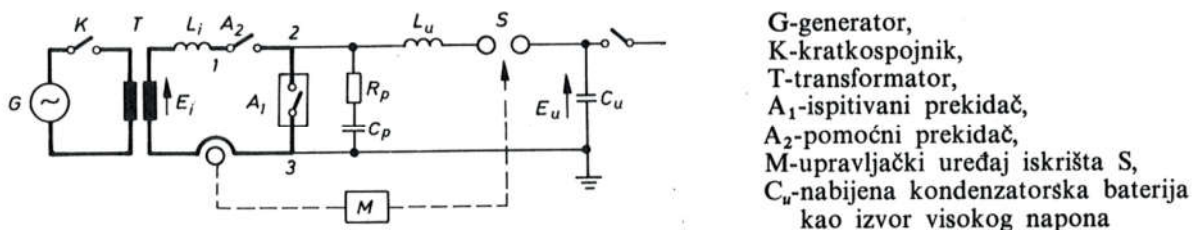
Sl. 773. Ispitni krug po metodi Weil-Dobke
