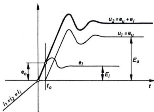
Sl. 777. Naponi i struje u krugu prema sl. 776.
