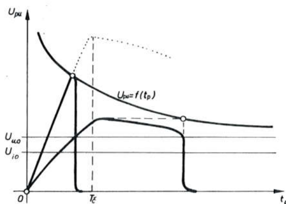
Sl. 406. Udarne karakteristika
