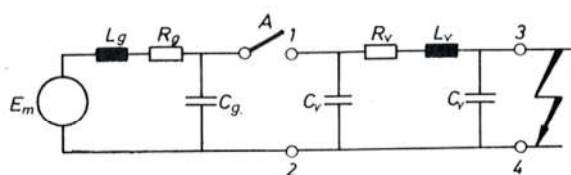
Sl. 6072. Nadomjesna shema titrajnog kruga
