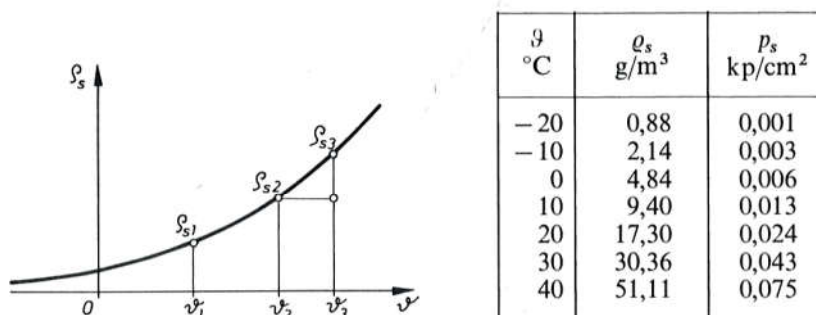
Sl. 746. Maksimalni sadržaj vodene pare u vlažnom zraku
