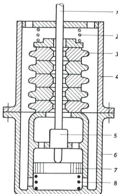
Sl. 731. Princip ekspanzijske komore s ubrizgavanjem tekućine
