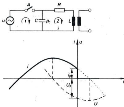
Sl. 6064. Naglo gašenje luka prije normalne nul-točke
