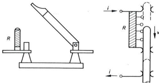
Sl. 701. Otporski prekidači
