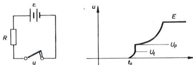
Sl. 6031. Promjena napona među kontaktima
