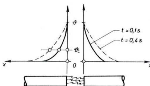
Sl. 318. Utjecaj električnog luka na temperaturu kontakta
