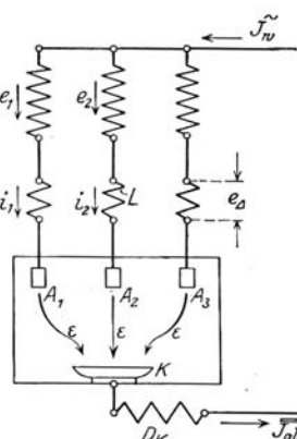
Abb. 232. Schaltskizze eines Großgleichrichters. D_K Kathodendrossel.
