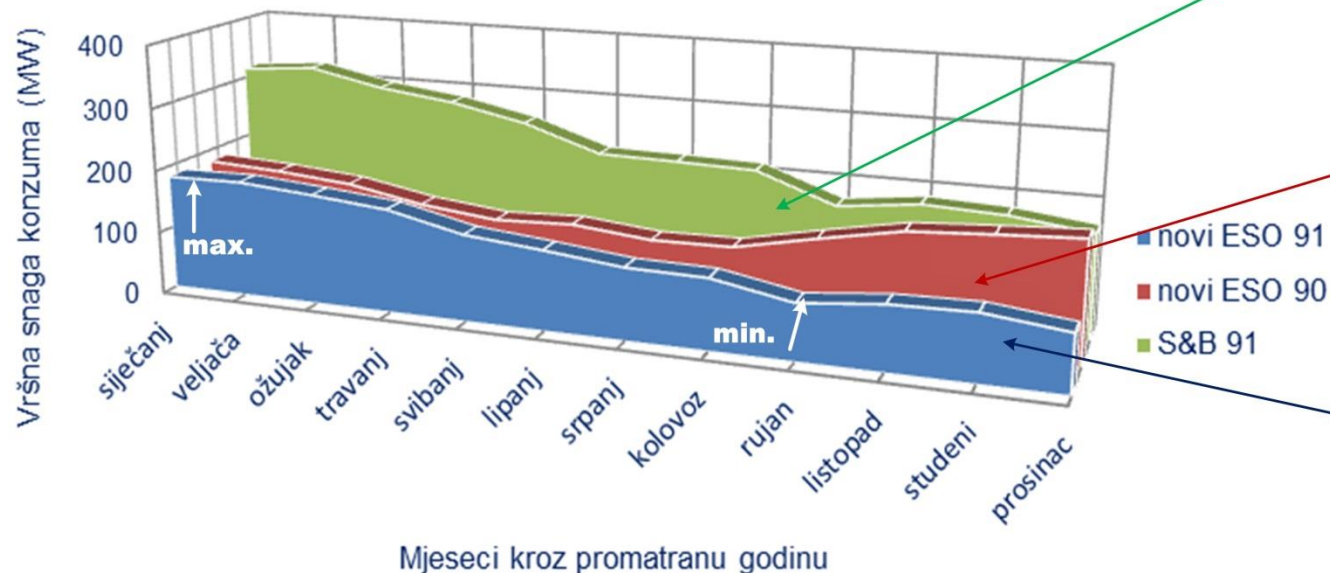
Tijek vrijednosti vršnog opterećenje potrošnje el. energije u distribucijskoj mreži 1990. i 1991. g. na području koje obuhvaća nova "Elektroslavonija"
