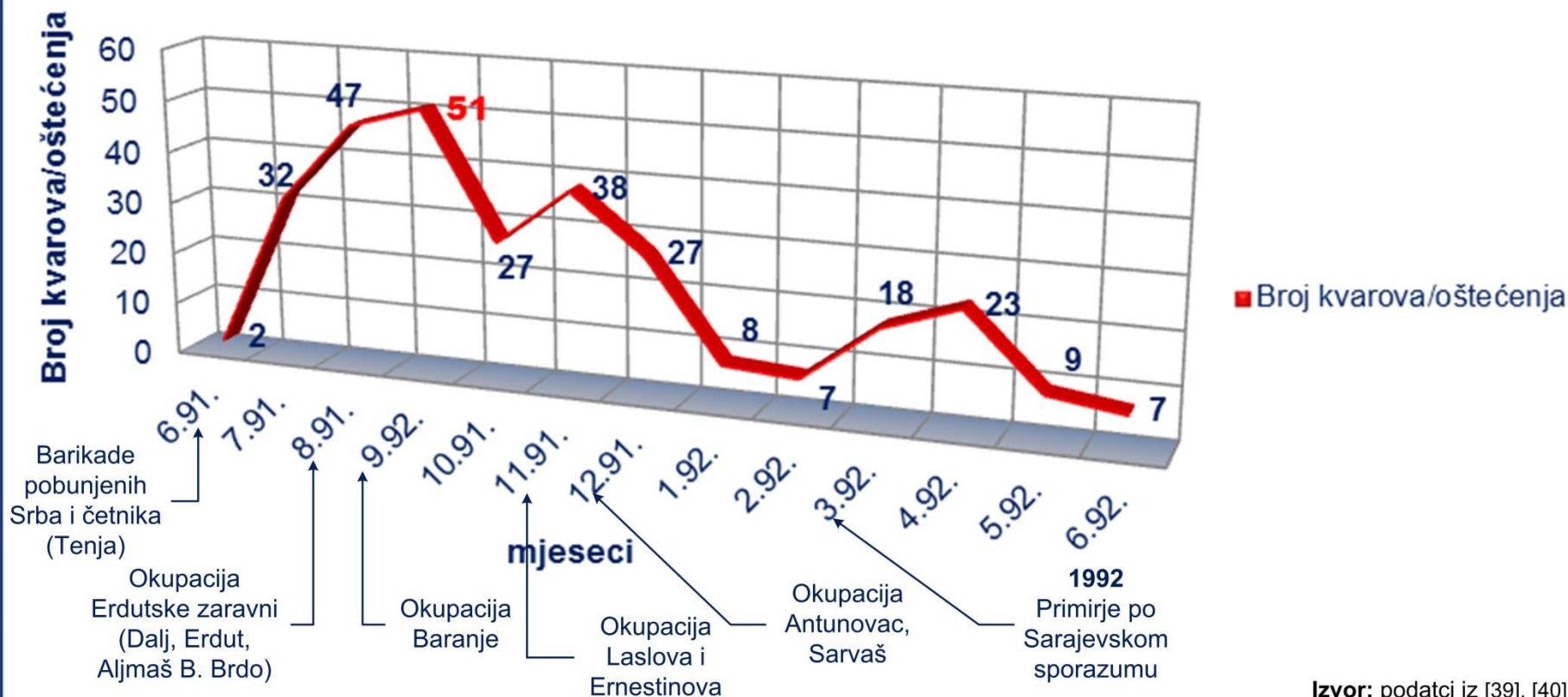
Broj kvarova/oštećenja u mreži 10 kV Elektroslavonije uslijed djelovanja neprijateljske artiljerije - PU Osijek
