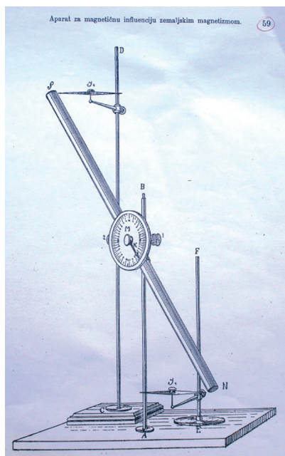
Sl. 11. Kučerin uređaj za magnetičnu influenciju zemaljskim magnetizmom
