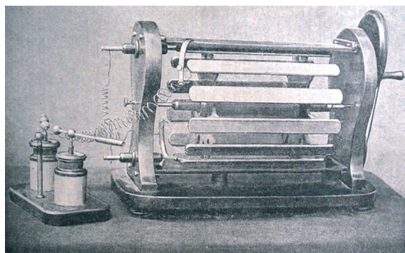
Sl. 14.: Pavlatov elektroforni uređaj
