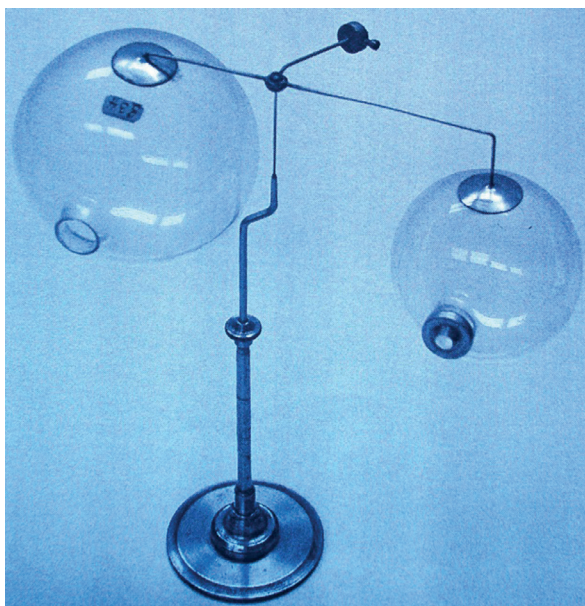
Sl. 8.: Dvořákov uređaj s Helmholtzovim rezonatorima
