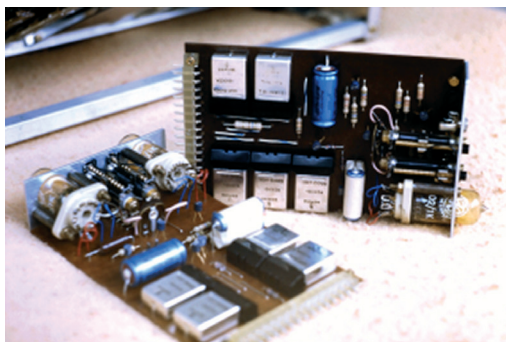
Sl. 8.: Prototipovi telegrafskih prijenosnika na ispitivanju
