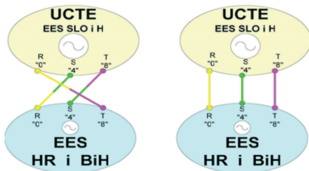
Sl. 12.: Sučelje ees-a Hrvatske i UCTE-a (ees-a SLO i H) prije (lijevo) i poslije (desno) usklađivanja redoslijeda faza
