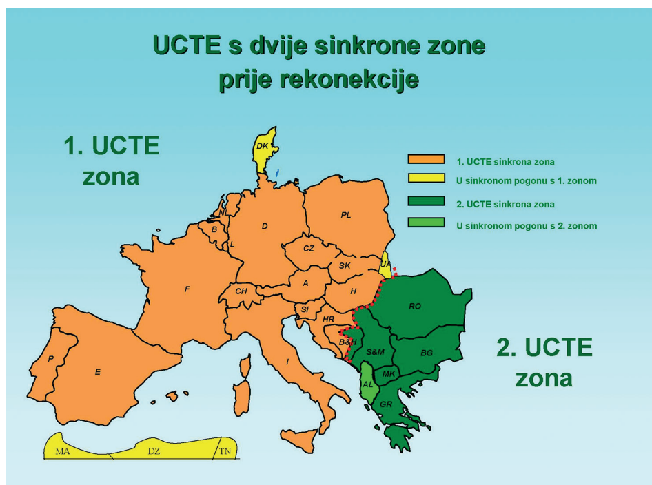
Sl. 5.: Interkonekcija UCTE sredinom 2004. godine (izvor: HEP – OPS)
