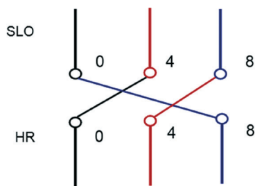
Sl. 10.: Principno predodžanje bivšeg stanja rasporeda faza na sučelju HR-SLO i HR-H ees-a
