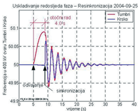
Sl. 17.: TS Tumbri – odziv frekvencije (izvor: IE, Institut za elektroprivredu)
