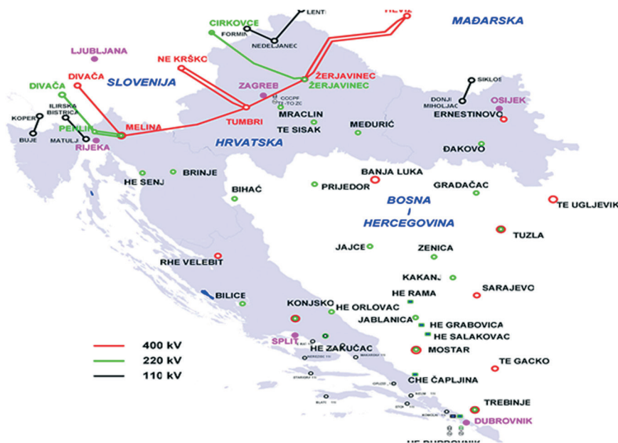
Sl. 14.: Spojni vodovi na sučelju ees-a Hrvatske i UCTE-a na kojima je proveden 'preplet' – usklađivanje redosljeda faza
