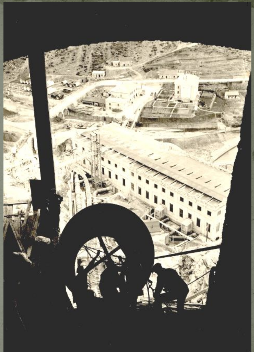
Transport dijelova tlačnih cjevoda prema vodnoj komori
