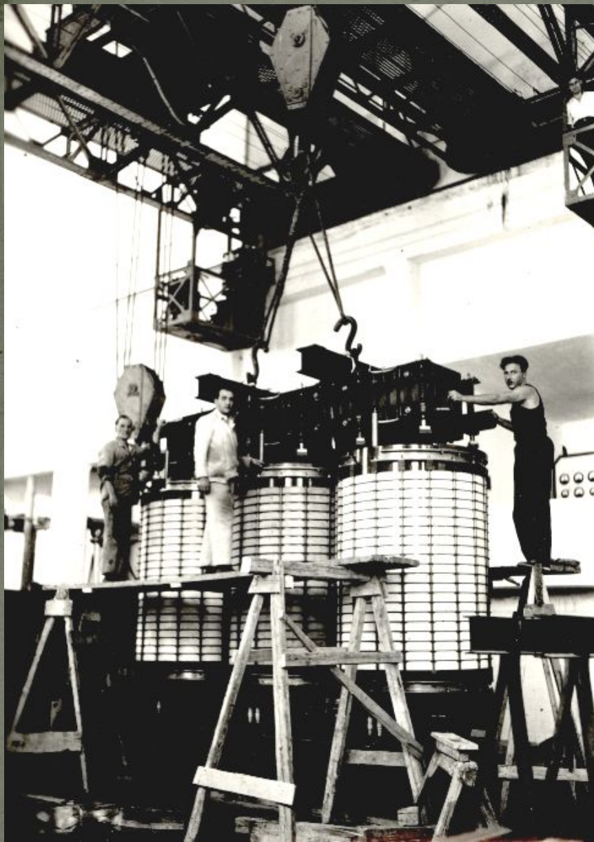
Montaža blok transformatora 42 MVA
