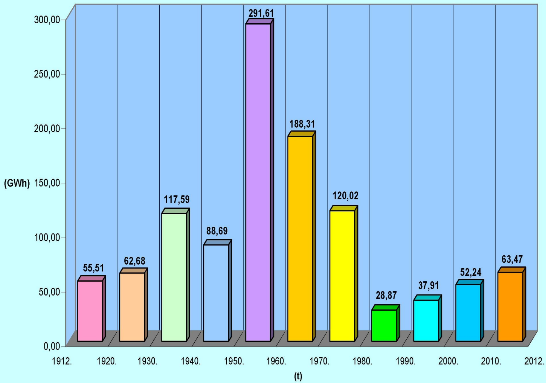
Srednja godišnja proizvodnja HE Kraljavec
