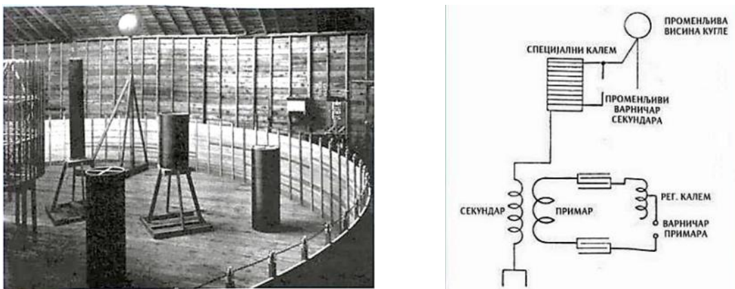
Slika 2 – Teslin ogroman tronamotni pojačavajući odašiljač i njegova shema [1]
