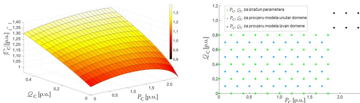
Slika 2. Trodimenzionalni prikaz domene i kodomene (rezolucija 0,1 p.u., nacrtano sa »surf« u Matlabu) te dvodimenzionalni prikaz vrijednosti domene
