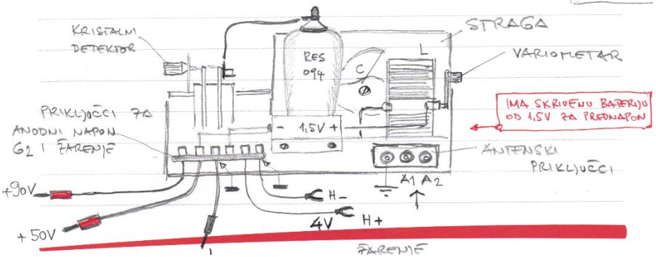
Sl. 5.: Skice iz tehničke dokumentacije prvog autora članka načinjena za refleksni jedno cijevni prijemnik s kristalnim detektorom
