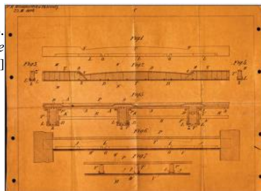
Slika 17. Tavanica izgrađena po Milankovićevom patentu [18]
