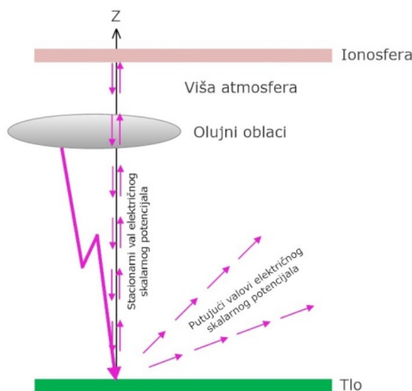
Slika 3 – Nastanak longitudinalnih putujućih skalarnih valova i "stupičastog" longitudinalnog stacionarnog vala električnog skalarnog potencijala
