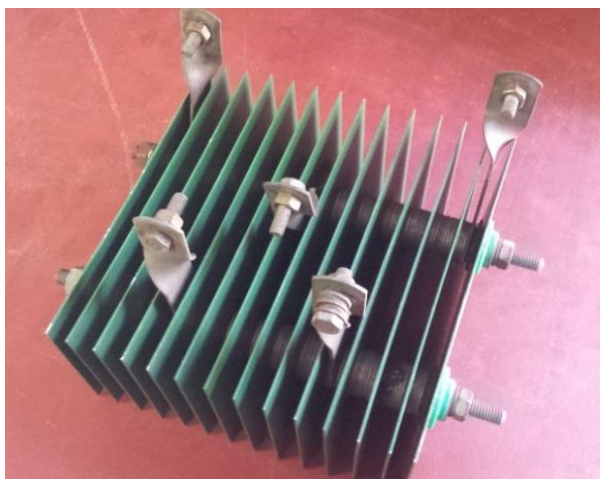
Slika 10. Selenski ispravljač tvrtke ISKRA. Očito se radi o ispravljaču u trofaznom mosnom spoju. U sredini su tri priključka za trofaznu mrežu, a na krajevima su dva priključka za istosmjerno trošilo.
