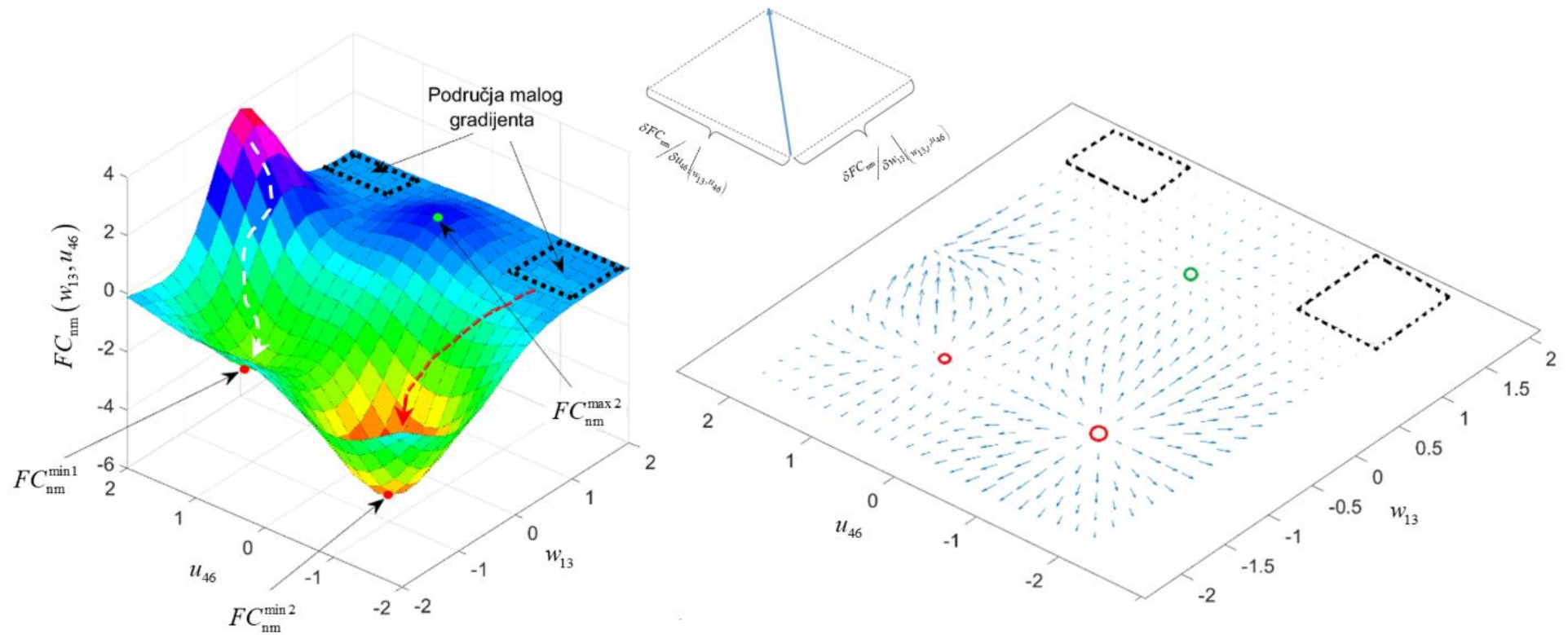
Slika 6. Trodimenzionalne grafički prikaz funkcije cilja FC_{nm}(u_{46}, w_{13}) s vektorima dvodimenzionalnog gradijenta funkcije u domeni (u_{46}-w_{13} ravnina), s dva optimizacijska puta do minimuma (crveni i bijeli isprekidani optimizacijski put)
