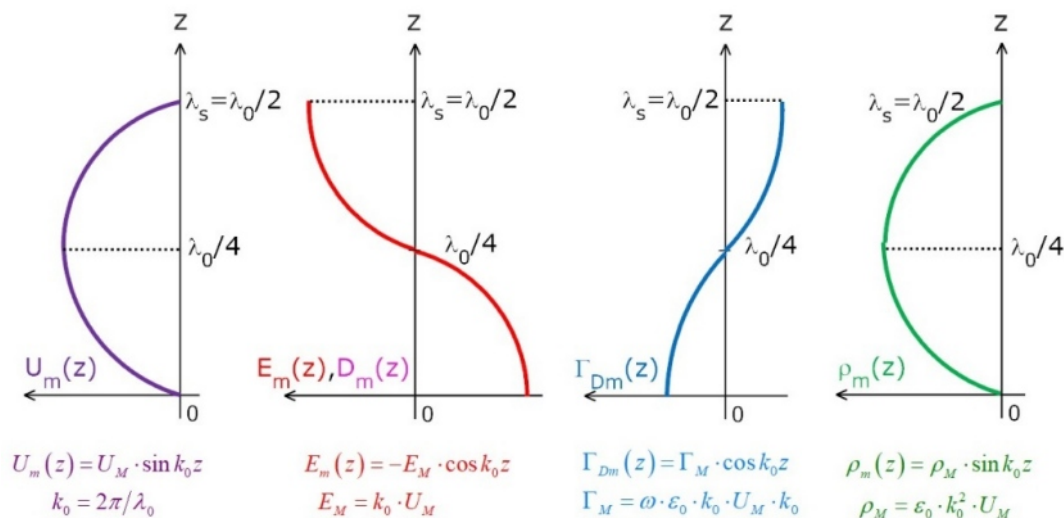
Slika 4 – Razdioba lokalnih amplituda U_m(z) , E_m(z) , \Gamma_{Dm}(z) i \rho_m(z) duž valne zrake u Teslinom longitudinalnom stacionarnom valu
