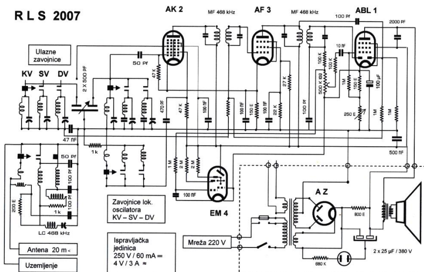
Sl. 11.: Savinov četverocijevni superheterodinski prijemnik sa zvučnikom
