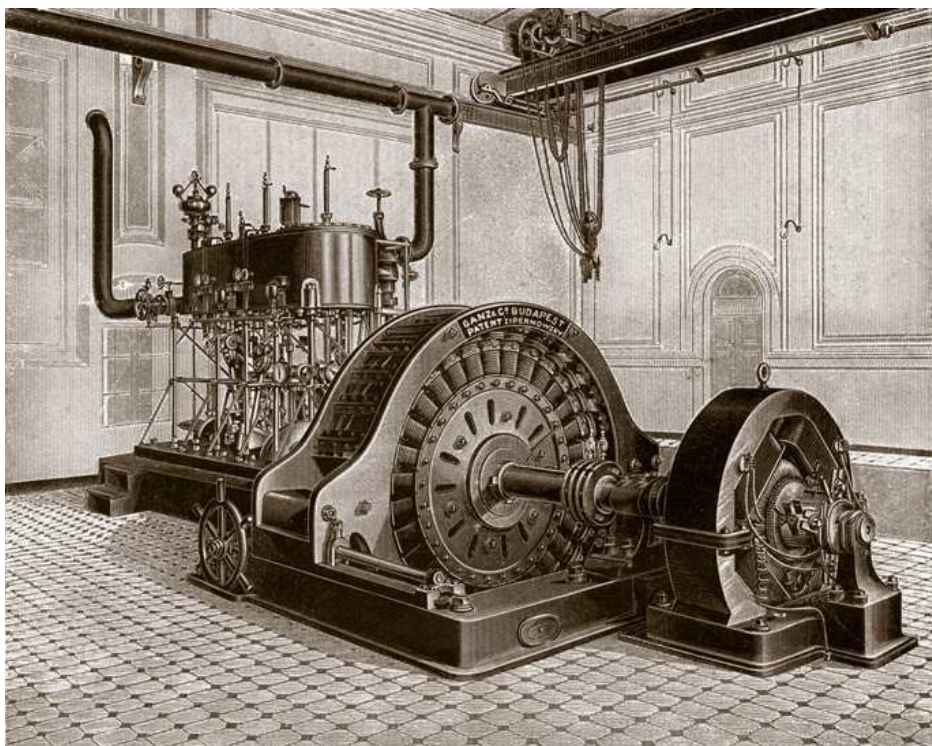
Sl. 4.: Jednofazni AC generator tipa A7 izravno spojen s parnim strojem i DC uzбудnikom (ranih 1890-ih godina) 44
