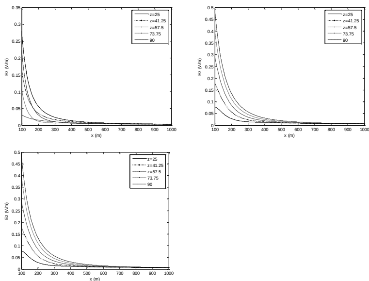
a) Monopol u slobodnom prostoru b) Monopol iznad idealno vodljive zemlje c) Monopol iznad konačno vodljive zemlje
