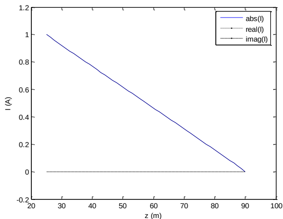
Sl. 6: Raspodjela struje inducirana duž vertikalnog monopola
