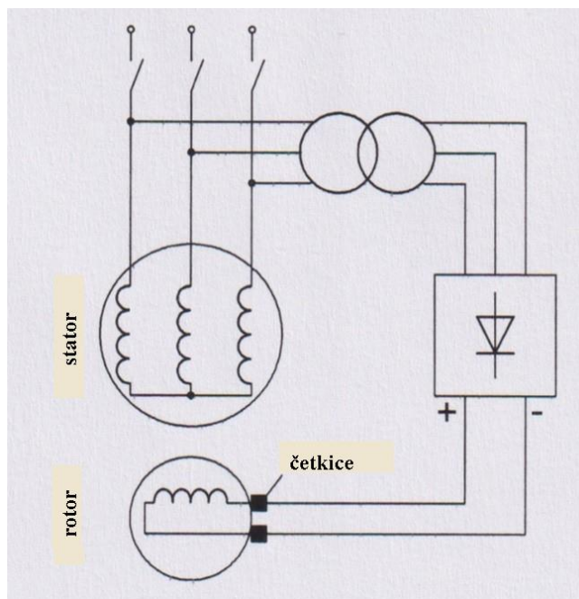
Slika 5. Načelna shema napajanja uzbude samouzbudnog generatora
