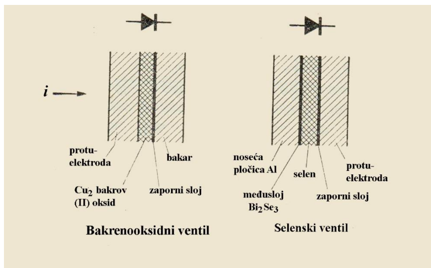
Slika 7. Usporedba slojevite strukture pločica bakrenooksidnog i selenskog električnog ventila
