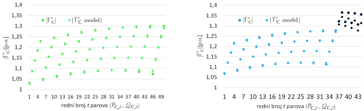
Slika 4. Izračunati potencijali Gaussovom metodom uspoređeni s izračunatim potencijalom regresijskim modelom uz iste ulaze (slika 2. desno s dosljedno korištenim bojama točaka t)
