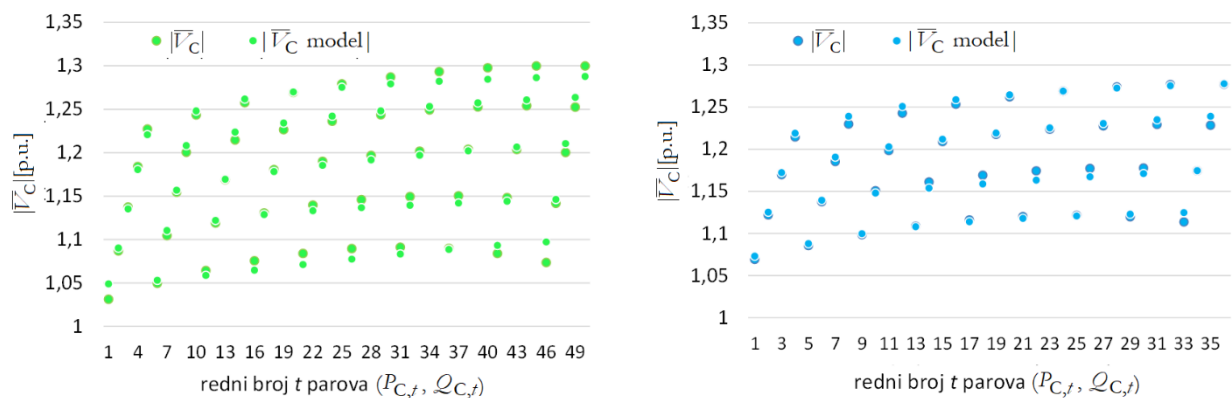
Slika 8. Ilustracija rezultata učenja na točkama za testiranje (zelene) i točkama za validaciju (plave) za dvije različito parametrirane mreže
