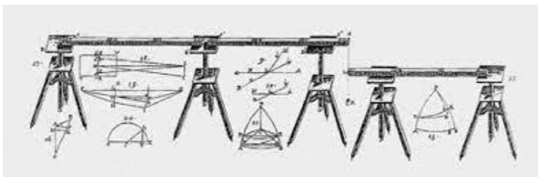
Sl. 10. Boškovićevi geodetski stalci i letve ([12], [32])
