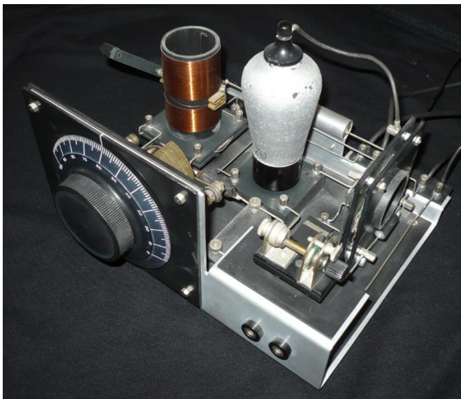
Sl. 4.: Prvi refleksni jednocijevni prijemnik s kristalnim detektorom Lovre Savina
