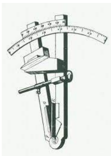
Sl. 5. Boškovićev vitrometar – druga inačica ([22], [24], [32])
