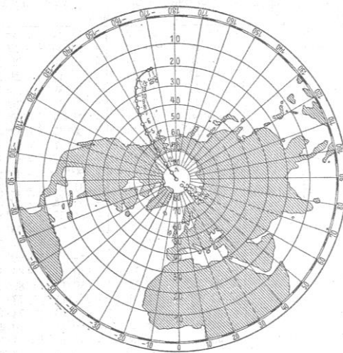
Slika 8. Sekularna putanja Zemljinog sjevernog rotacijskog pola prema izračunu Milutina Milankovića Izvor: [8]
