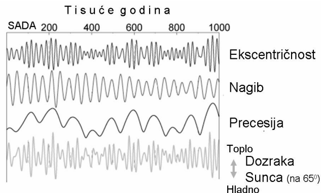
Slika 5. Učinak Milankovićevih ciklusa na osunčavanje Zemlje Izvor: [3]
