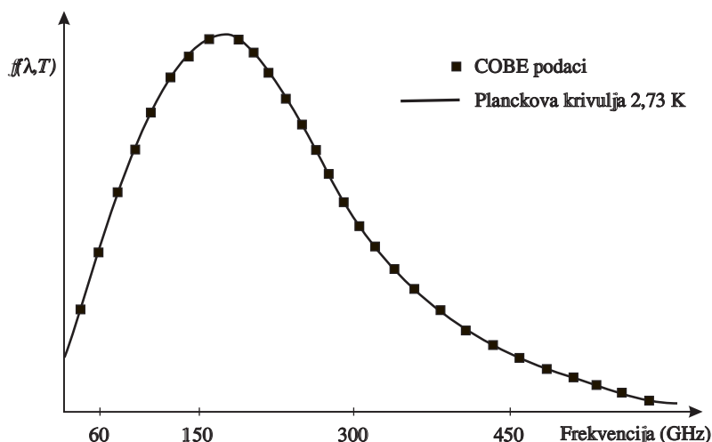
Slika dD1.4- Spektralna gustoća mikrovalnog pozadinskog kozmičkog zračenja: teorijska krivulja i eksperimentalni podatci.
