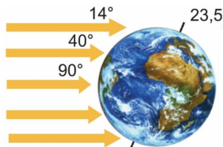
Slika 3. Kut pada sunčevih zraka na površinu Zemlje Izvor: [2]
