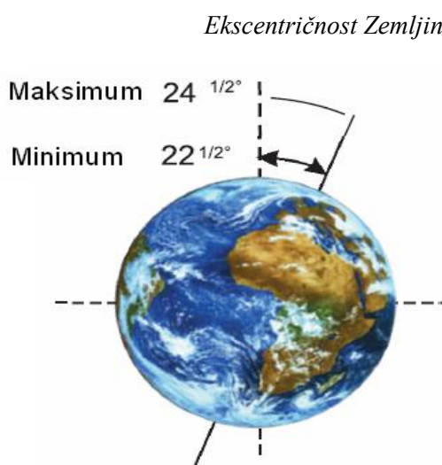
Slika 2 Promjena nagiba Zemljine osi rotacije u odnosu na ravan orbite Izvor: [2]
