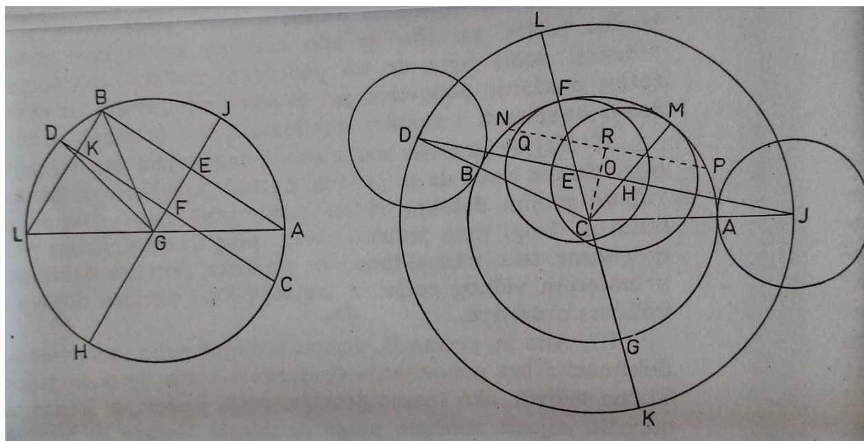
Sl.1. Kružni mikrometar – Načela mjerenja u vidnom polju ([19], [32])
