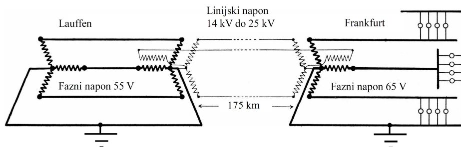
Sl. 11. Trofazni AC prijenosni sustav Lauffen-Frankfurt 184
