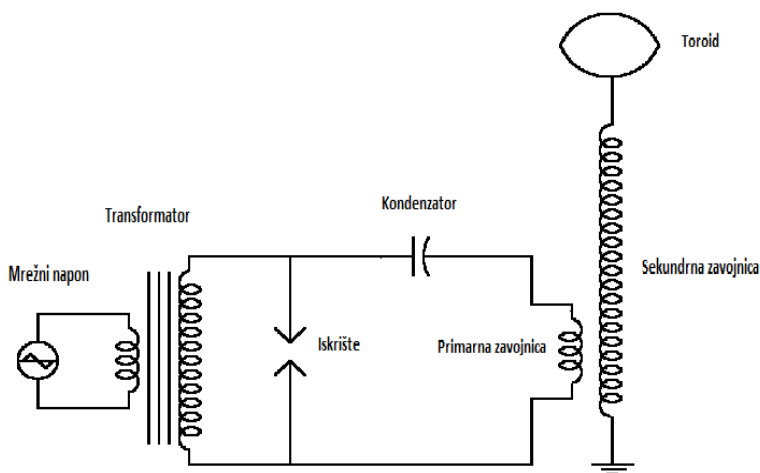
Sl. 1: Osnovna shema Teslinog uređaja
