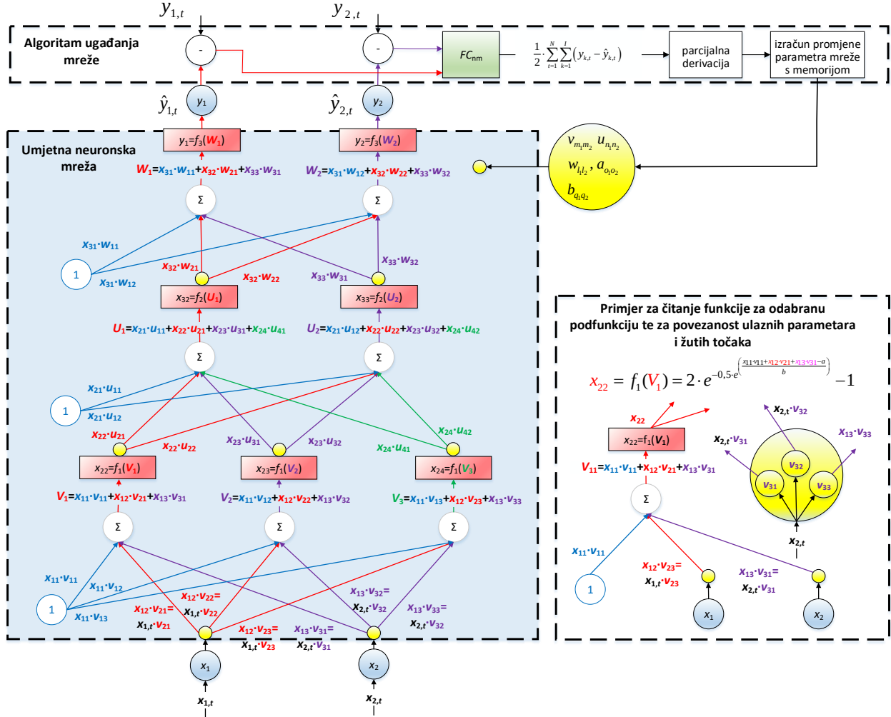
Slika 5. Primjer umjetne neuronske mreže s tri sloja podfunkcija (prvi s tri podfunkcije, drugi i treći s dvije podfunkcije), dva ulaza u mrežu i dva izlaza iz mreže s dijelom za ugađanje parametara
