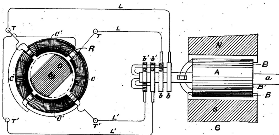
Sl. 3.: Dvofazni AC prijenosni sustav - dvofazni sinkroni AC generator i dvofazni sinkroni AC motor iz Teslinog američkog patenta br. 382.280
