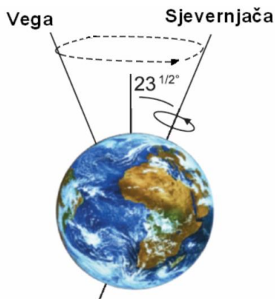
Slika 4. Revolucija Zemljine rotacijske osi Izvor: [2]
