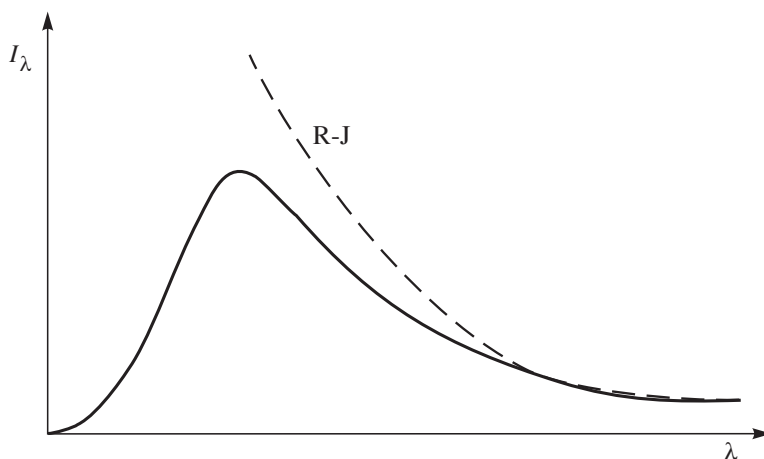
Slika 2.2 - Spektralna gustoća zračenja i Rayleigh-Jeansov zakon
