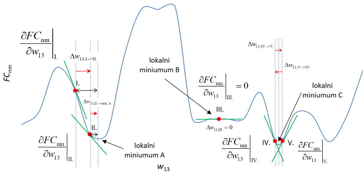
Slika 7. Ilustracija modela za promjenu parametara neuronske mreže
