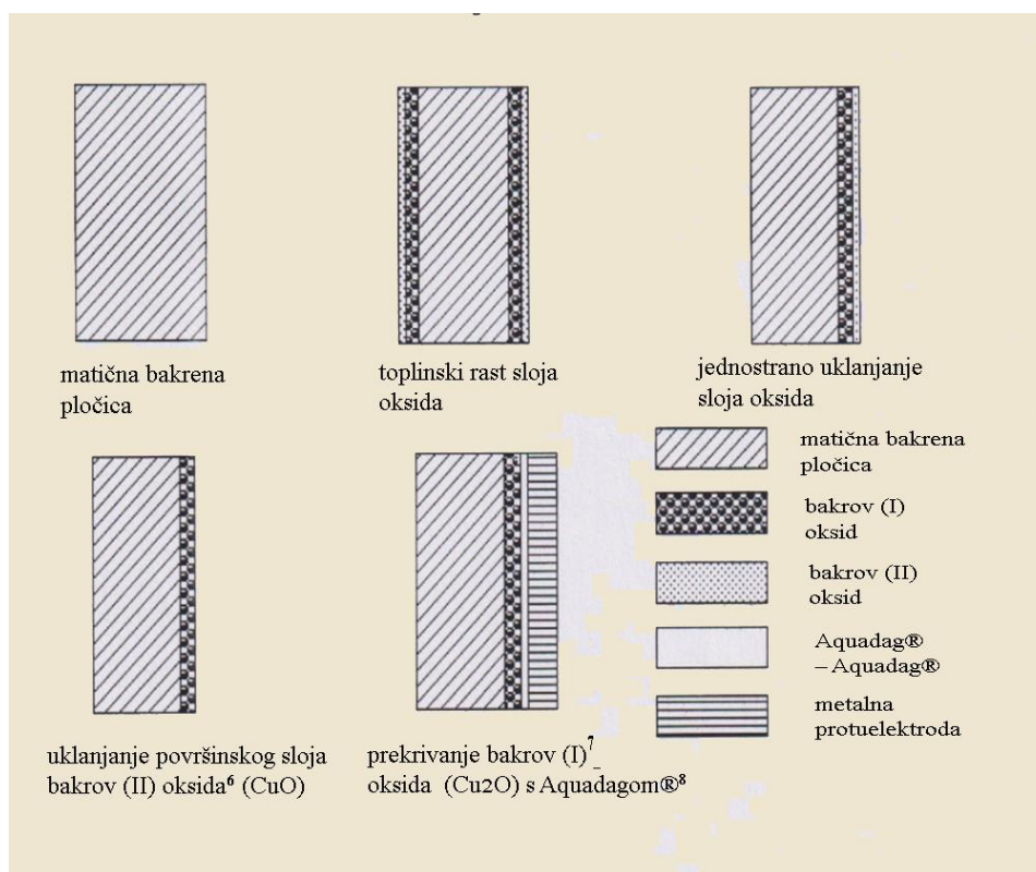
Slika 8. Faze izrade bakrenooksidnog ventila
