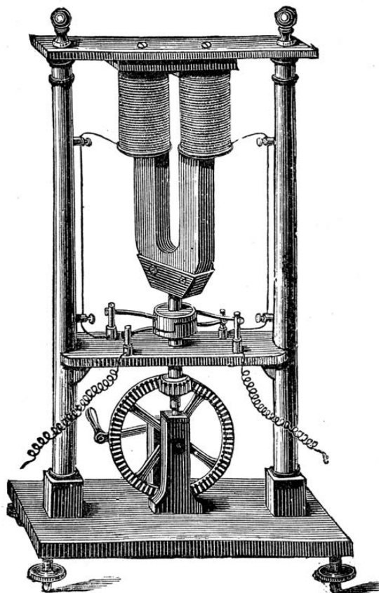
Sl. 2.: Skica Pixijevog jednofaznog AC generatora
