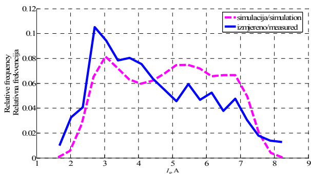
Slika 9. Razdioba vrijednosti tjedne krivulje 5. strujnog harmonika na TS 10/0,4 kV TS B. Magovca 44
