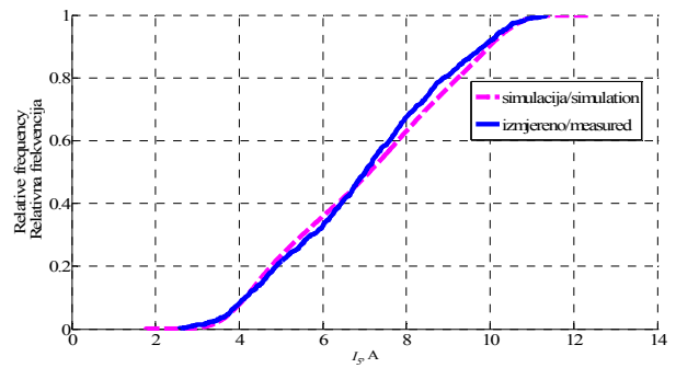
Slika 8. Razdioba vrijednosti tjedne krivulje 5. strujnog harmonika na TS 10/0,4 kV TS B. Magovca 38
