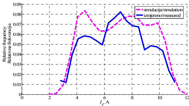
Slika 8. Razdioba vrijednosti tjedne krivulje 5. strujnog harmonika na TS 10/0,4 kV TS B. Magovca 38
