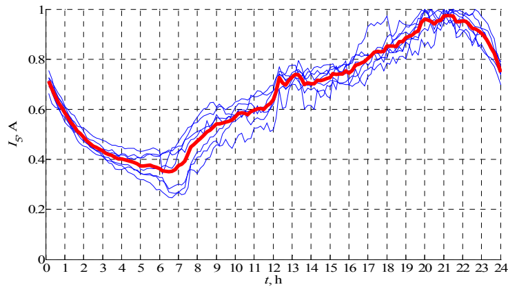
Slika 4. Normirane prosječne dnevne krivulje 5. harmonika struja i pripadajući centroid klastera 1
