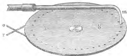
Sl. 37. Sirena po Tyndallu.
