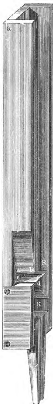
Sl. 61. Obična svirala.
