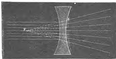
Sl. 125. Put zrakâ u ugnutoj leći.
