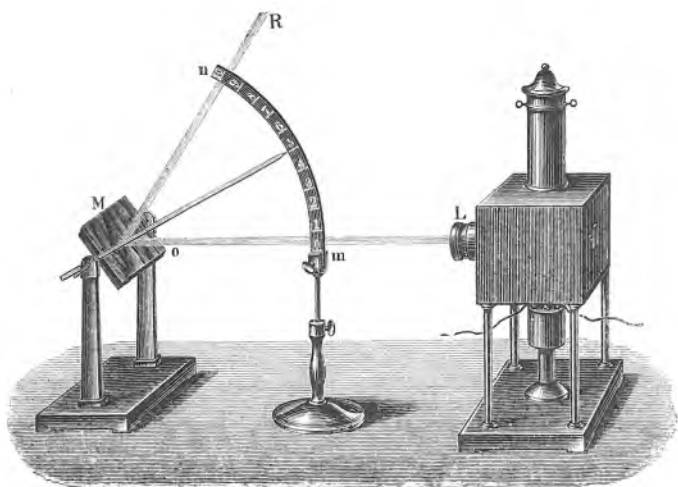
Sl. 95. Odbijanje svjetlosti.
