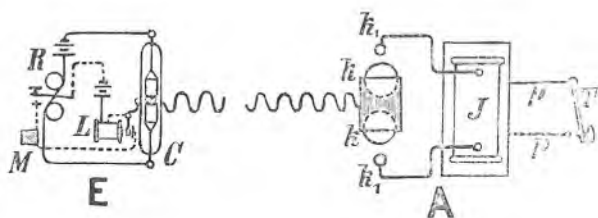
Sl. 228. Telegrafovanje bez žica.
