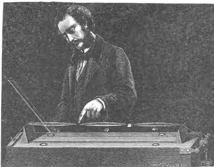
Sl. 45. Njihanje žice; čvorovi i trbušci.
