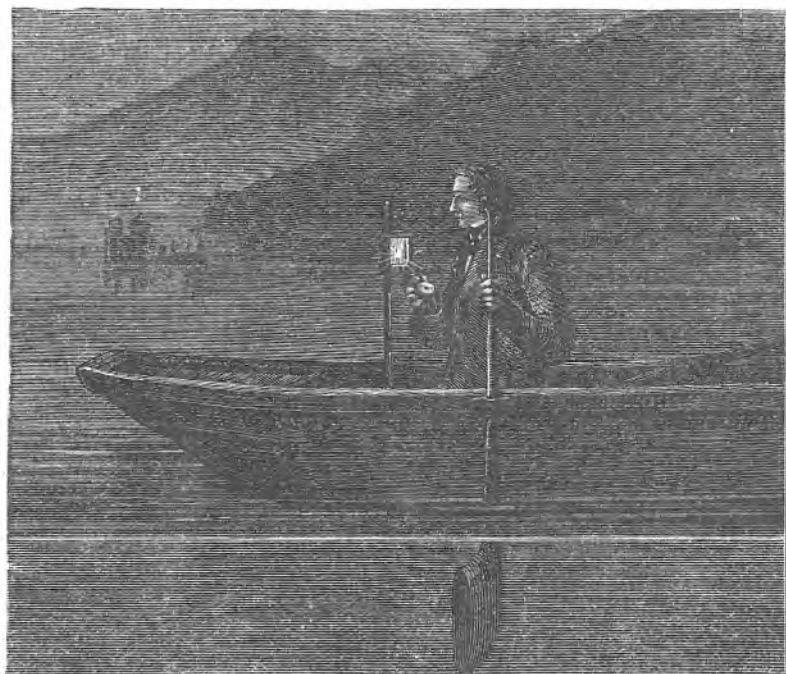
Sl. 35. Mjerenje brzine zvuka u vodi.
