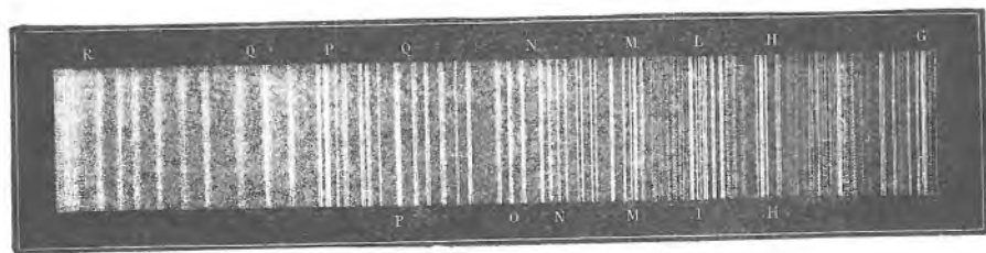
Sl. 172. Dio ljubičastoga i ultraljubičastoga spektra sunčanoga.
