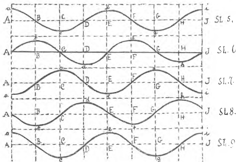
Sl. 5—9. Oblik uztalasane vode.
