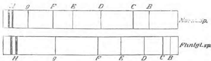
Sl. 166. Prizmatički i normalni spektar.
