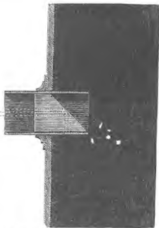
Sl. 117. Prizma za totalnu refleksiju.
