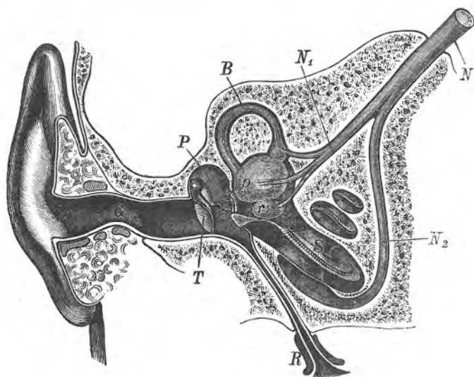
Sl. 77. Prosjek kroz uho.
