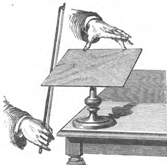
Sl. 56. Titranje ploče.
