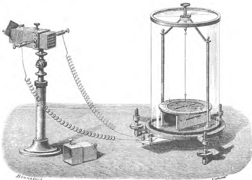
Sl. 171. Nobilijev termo-multiplikator.
