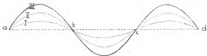
Sl. 20. Ukrštavanje (interferencija) dvaju valova.
