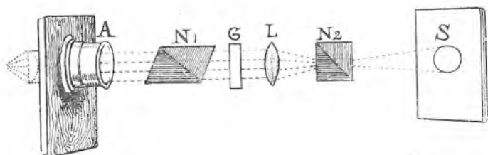
Sl. 213. Pločica sadre u polarizovanoj svjetlosti.
