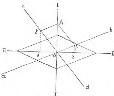
Sl. 211. Pločica sadre među ukrštenim nikolima.
