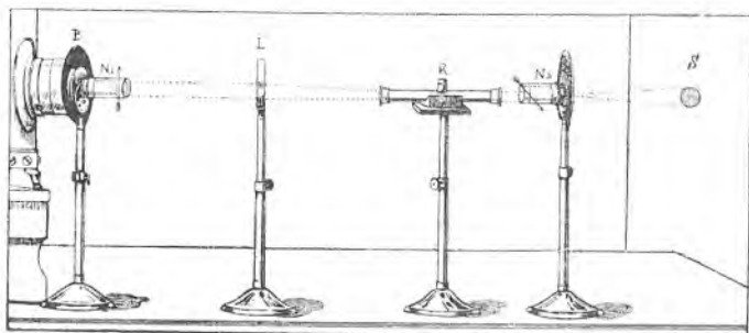
Sl. 204. Zakretanje smjera titranja u polarizovanoj svjetlosti.
