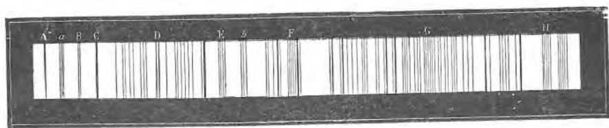
Sl. 146. Spektar Sunca s Fraunhoferovim crtama.
