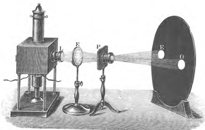
Sl. 190. Dvostruko lomljenje svjetlosti u islandskom dvolomcu.
