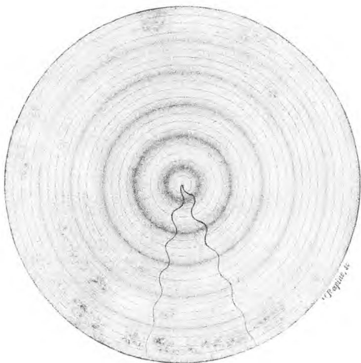
Sl. 22. Rasprostiranje zvučnoga vala u uzduhu.
