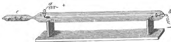
Sl. 214. Fosforesciranje stakla od katodnih zraka.
