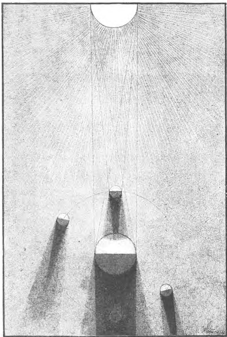
Sl. 94. Pomrčine Sunca i Mjeseca.
