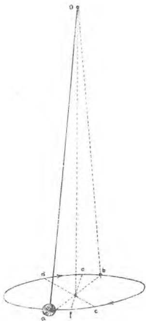
Sl. 202. Sastavljanje njihaja.
