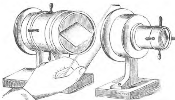
Sl. 206. Pločica tinjca medju nikolima.
