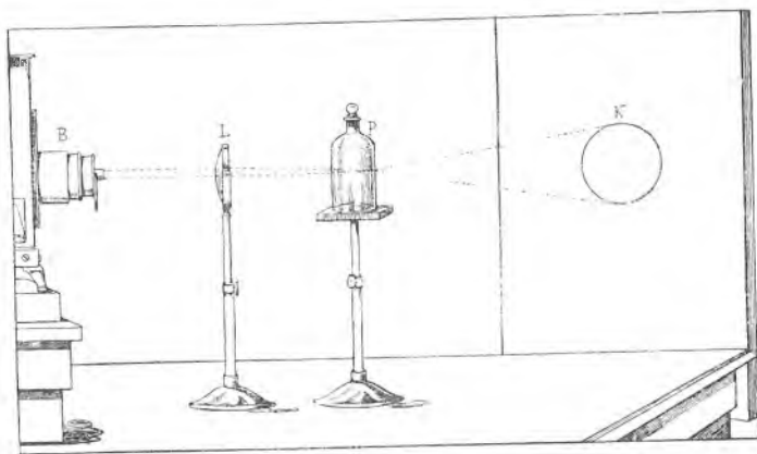
Sl. 173. Petrolej fluorescira.
