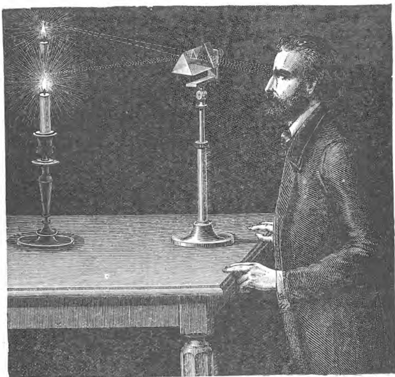
Sl. 121. Slika svijeće kroz prizmu.
