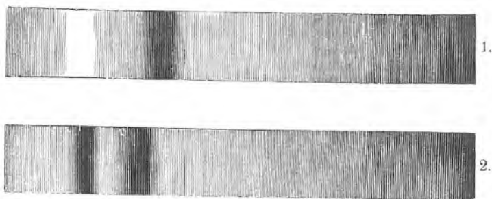
Sl. 147. Spektar apsorpcije crvene boje magenta (1) i krvi (2).
