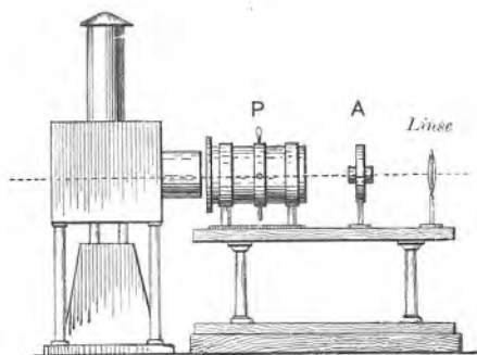
Sl. 193. Valovi svjetlosti polarizovani pomoću dvaju nikola.
