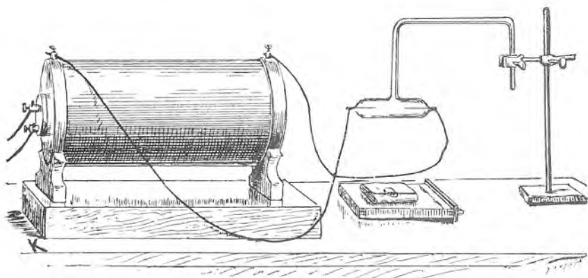
Sl. 221. Fotografovanje pomoću Röntgenovih zrakā.
