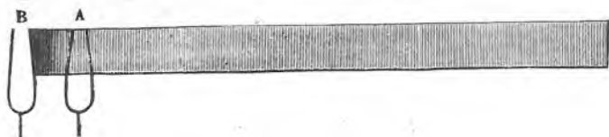
Sl. 80. Uništavanje zvuka.
