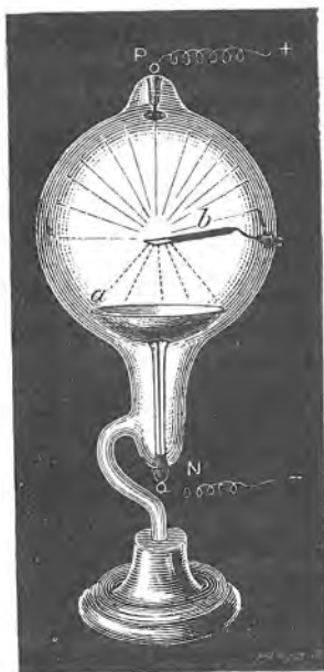
Sl. 219. Katodne zrake razvijaju toplinu.
