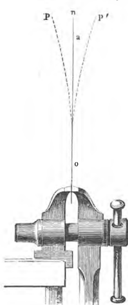
Sl. 48. Njihanje šipke učvršćene na jednom kraju.
