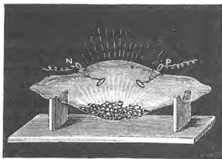
Sl. 216. Fosforesciranje rubina od katodnih zraka.
