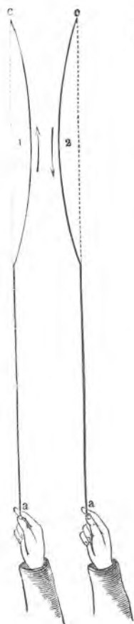
Sl. 15. Odbijanje vala.
