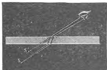
Sl. 118. Lomljenje u staklenoj ploči.
