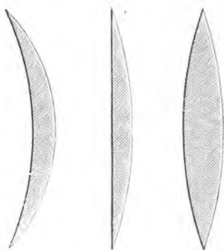
Sl. 122. Pupčaste leće (leće sabirajuće).
