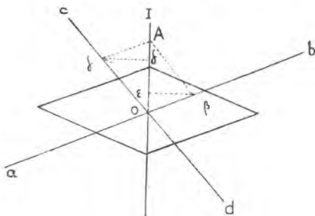
Sl. 212. Pločica sadre među usporednim nikolima.
