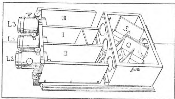
Sl. 138. Aparat za miješanje boja.
