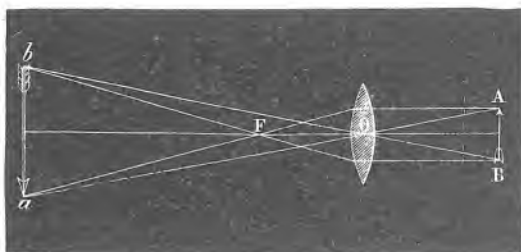
Sl. 128. Kako postaje slika u leći sabirači.
