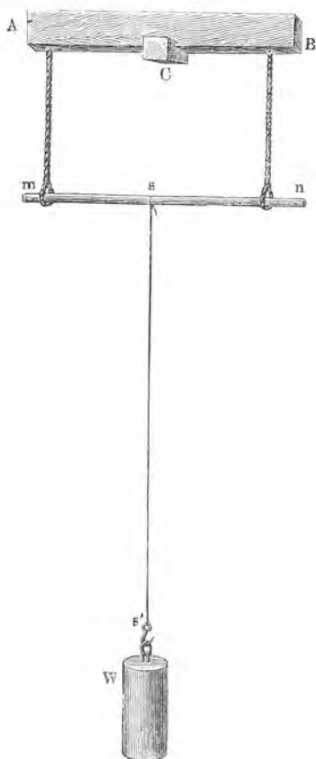
Sl. 41. Titranje napete žice u uzduhu.
