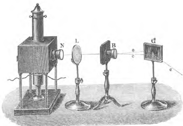
Sl. 201. Ravno zrcalo prepoznaje polarizovanu svjetlost.
