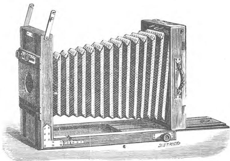
Sl. 175a. Fotografijska kamera (otvorena).
