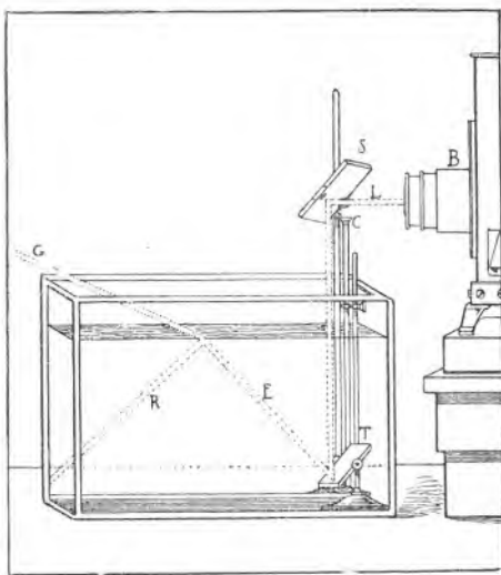
Sl. 115. Totalna refleksija.
