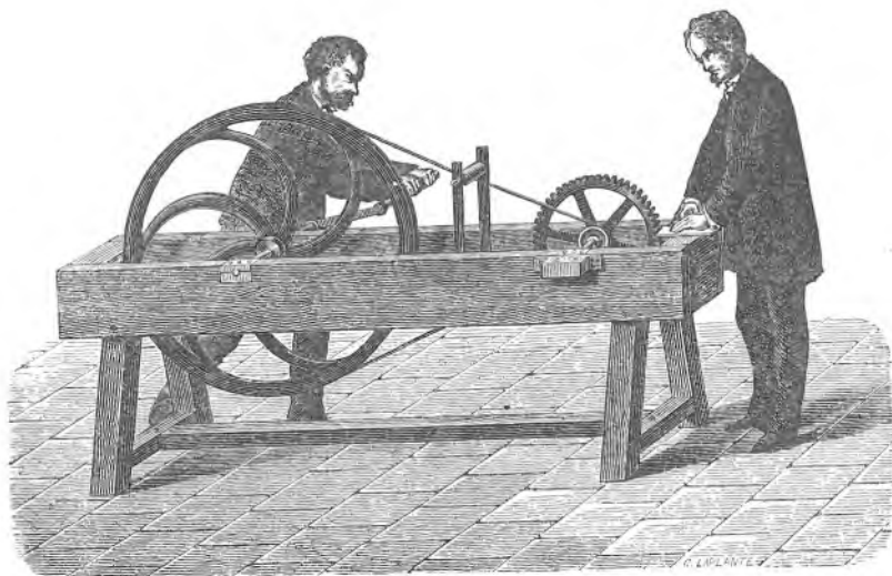
Sl. 36. Savartovo zubato kolo.
