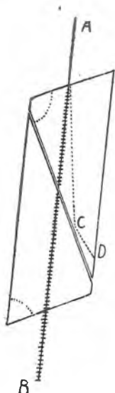
Sl. 191. Nikolov bridnjak ili kraće „nikol“.
