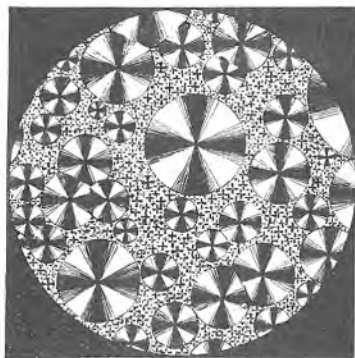
Sl. 209. Slike salacine u polarizovanoj svjetlosti.
