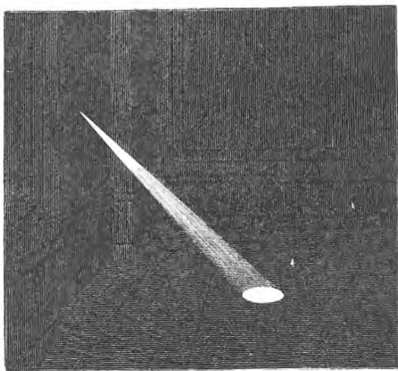
Sl. 84. Pramen sunčane svjetlosti u tamnoj sobi.
