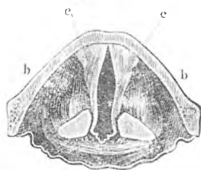
Sl. 68. Organ govora.
