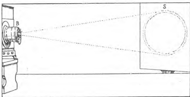
Sl. 87. Zrake svjetlosti iz jedne točke jesu divergentne (razilaze se).
