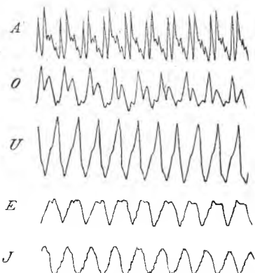
Sl. 76. Fonografske krivulje.
