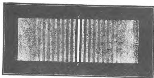
Sl. 162. Pruge interferencije (ukršćavanja).
