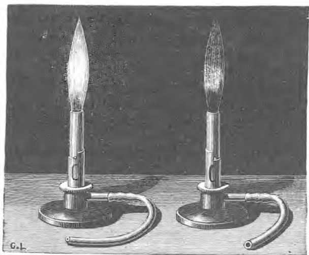
1. Sl. 139. Bunsenov plamenik: 2. 1. svijetao i manje topao plamen; 2. manje svijetao i već vruć plamen.
