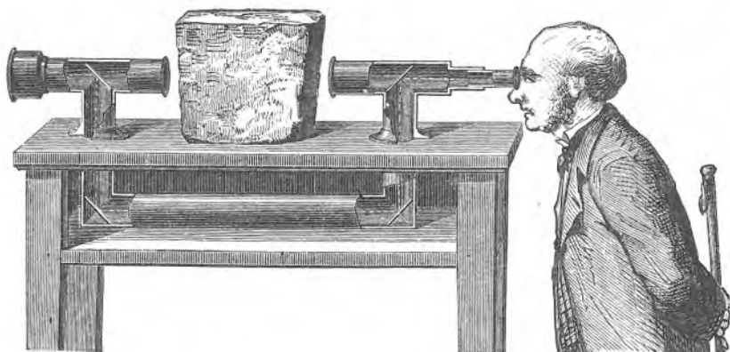
Sl. 101. Magičan durbin.
