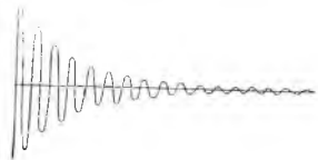
Sl. 182. Utišavanje titraja.
