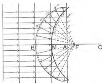
Sl. 150. Odbijanje svjetlosti od pupčastog zrcala.
