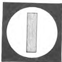
Sl. 196. Pločica turmalina u okviru.
