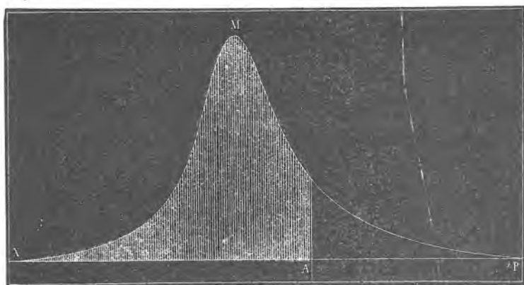
Sl. 168. Krivulja za zrake topline u spektru.
