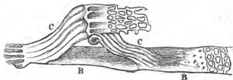
Sl. 78. Cortijev organ.
