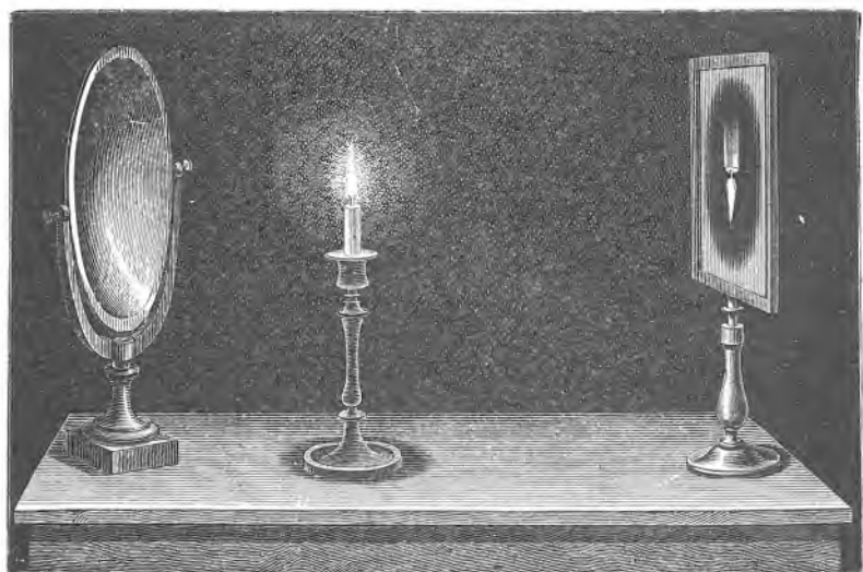
Sl. 103. Ugnuto zrcalo; obrnuta i uvecana slika predmeta.
