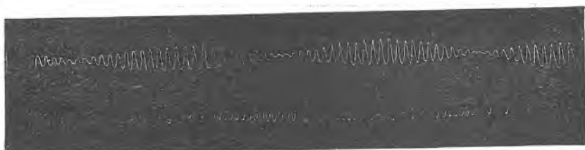
Sl. 82. Treptanje tonova.
