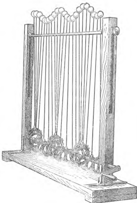
Sl. 4. Model valovitoga gibanja.
