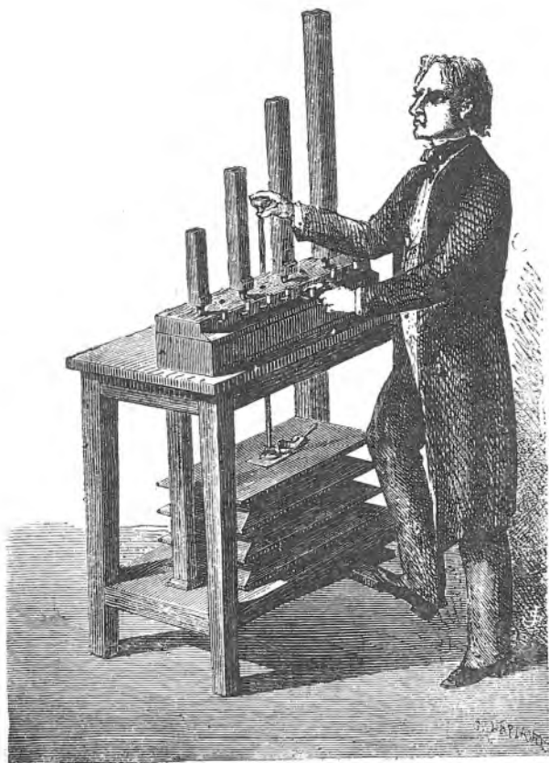
Sl. 65. Zakon za svirale.
