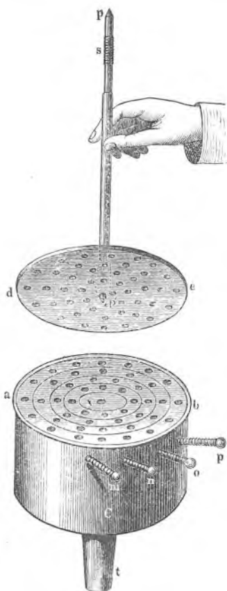
Sl. 38. Doveova sirena.
