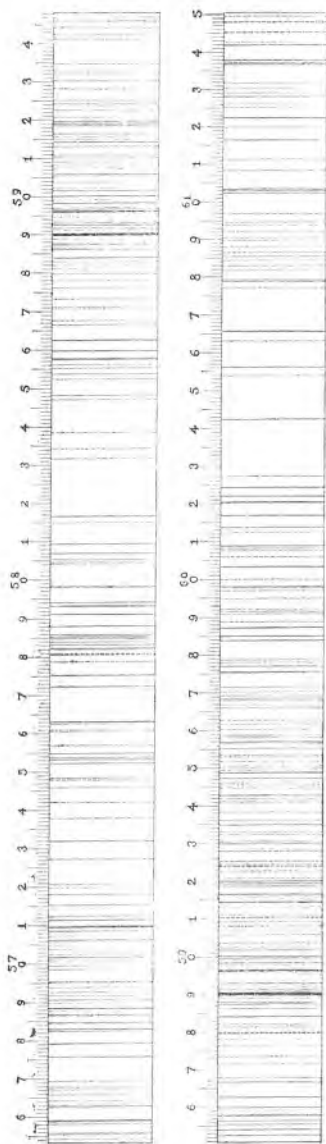
St. 167. Fotografija spektra.
