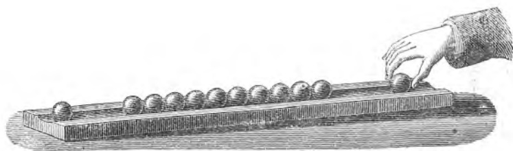
Sl. 11. Uzdužno titranje.
