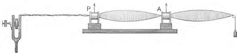
Sl. 186. Propuštanje polarizovana vala.
