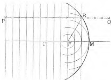
Sl. 152. Odbijanje ravna vala od ugnuta zrcala.
