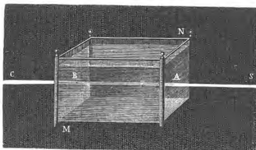
Sl. 109. Lomljenje svjetlosti.
