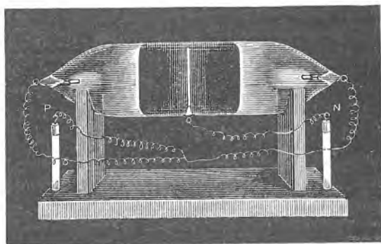
Sl. 215. „Tamni prostor“ katodnih zraka.
