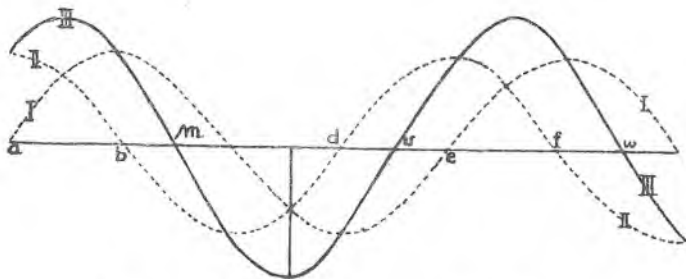
Sl. 19. Ukrštavanje (interferencija) dvaju valova.
