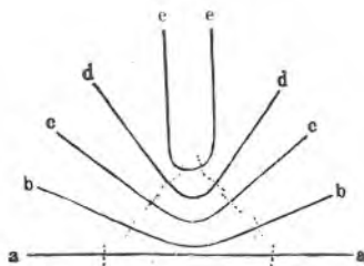
Sl. 52. Njihanje akustične šipke.
