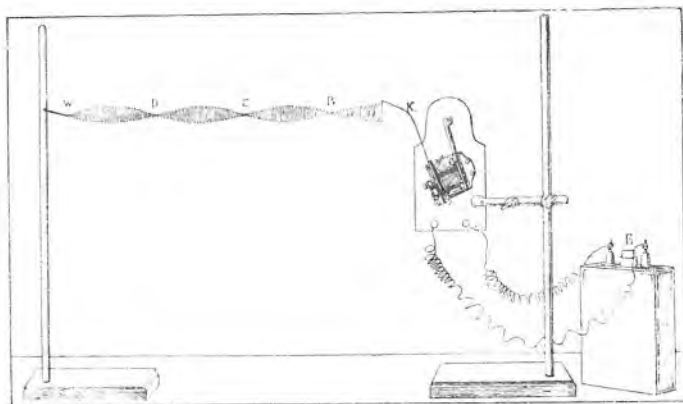
Sl 179. Princip Lippmannova fotografovanja u prirodnim bojama.
