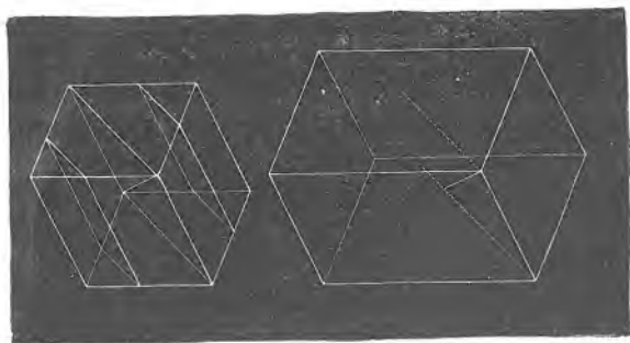
Sl. 189. Romboedri islandskoga dvolomeca.
