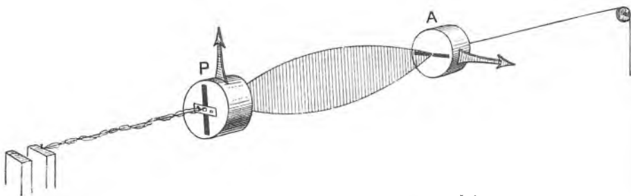
Sl. 187. Uništavanje polarizovana vala na užetu.
