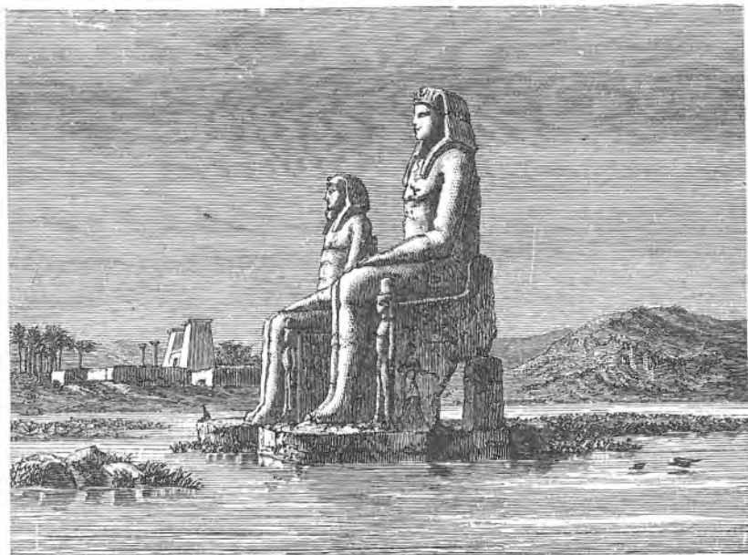
Sl. 46. Memnonovi kipovi.
