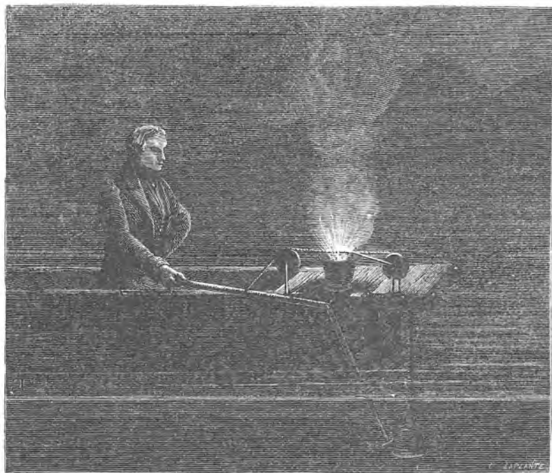
Sl. 34. Mjerenje brzine zvuka u vodi.
