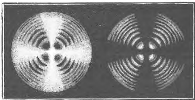
Sl. 208. Obojeni krugovi s krstom u polarizovanoj svjetlosti.
