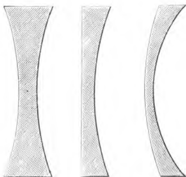
Sl. 123. Ugnute leće (leće rastresajuće).
