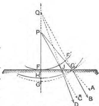
Sl. 154. Lomljenje valova svjetlosti.
