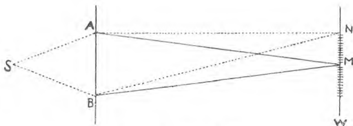
Sl. 161. Youngov pokus.
