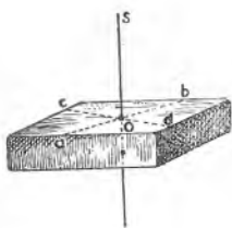
Sl. 210. Pločica sadre.
