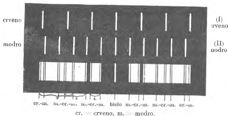
Sl. 165. Skretanje svjetlosti u Nobertovoj mrežici.
