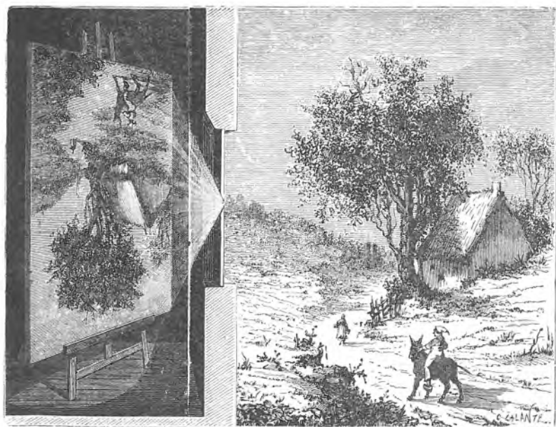
Sl. 93. Slika kraja u tamnoj sobi (camera obscura).
