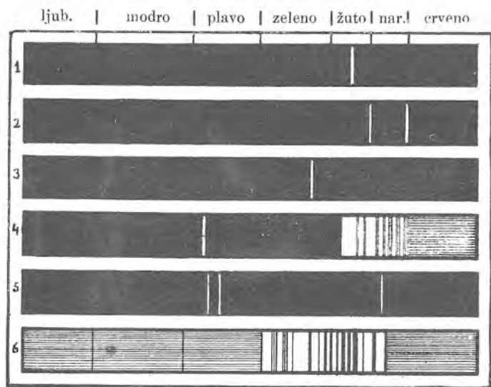
Sl. 140. Spektri različitih tvari.
