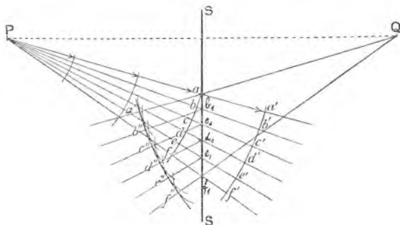
Sl. 16a. Odbijanje vala.
