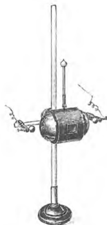
Sl. 225. Righijev oscilator.
