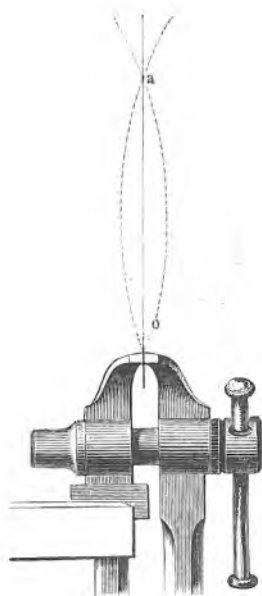
Sl. 49. Njihanje šipke utišane.
