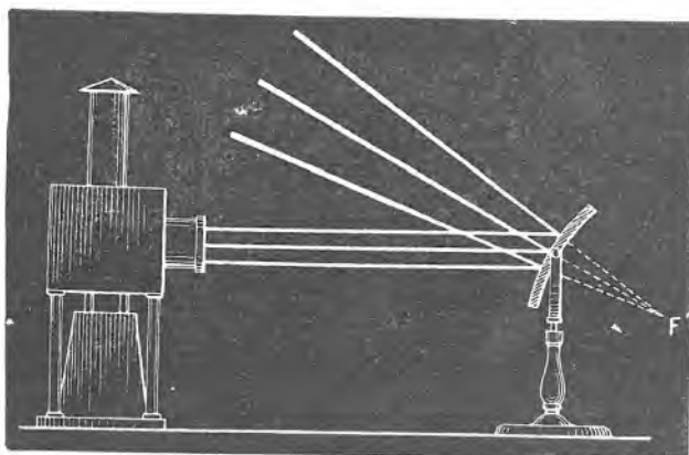
Sl. 151. Odbijanje svjetlosti od pupčasta zrcala.
