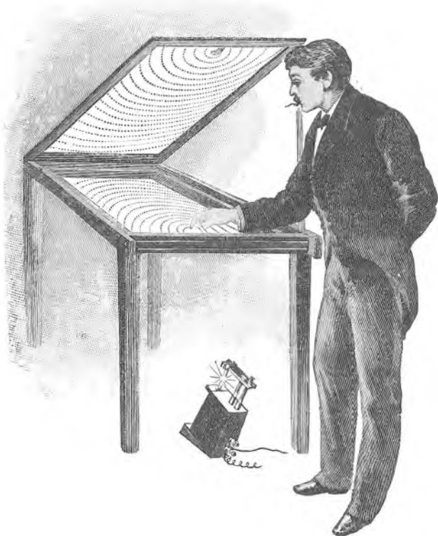
Sl. 3. Žlijeb za valove.
