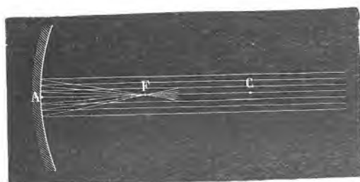
Sl. 105. Glavno žarište ugnuta zrcala.
