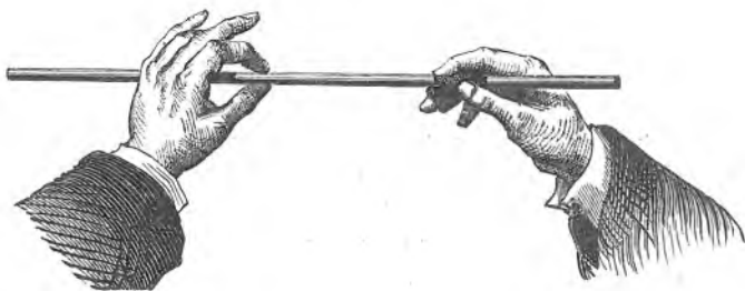
Sl. 59a. Titranje uzdužno štapom.
