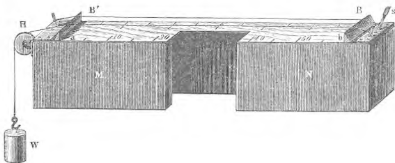
Sl. 40. Monokord ili sonometar.
