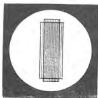
Sl. 197. Dvije pločice turmalina u usporednu položaju.
