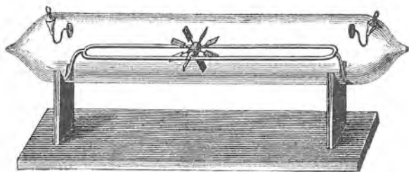
Si. 217. Mehanično djelovanje katodnih zraka.
