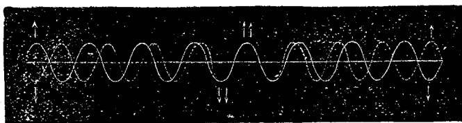
Sl. 81. Ukrštavanje valova nejednake dužine.
